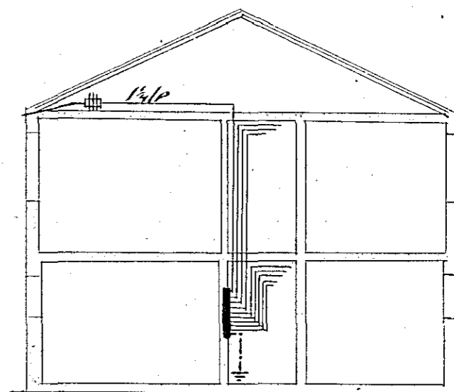
Skurður
