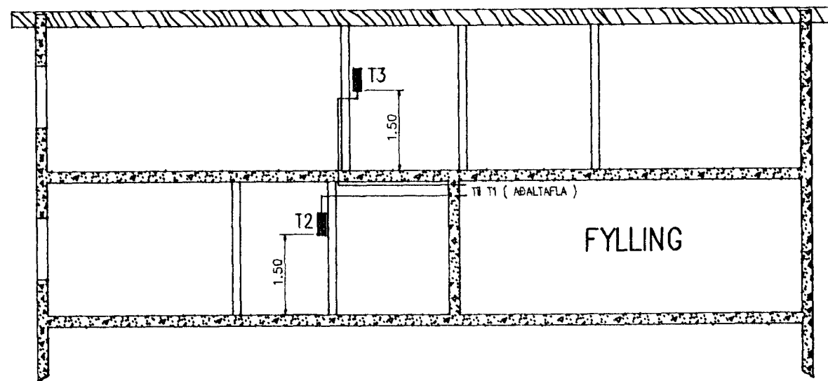
Sniðmynd B Mkv. 1:100
