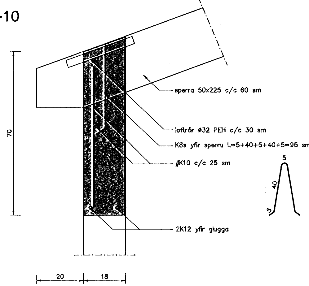
Snið 15-15 Mkv. 1 : 10
