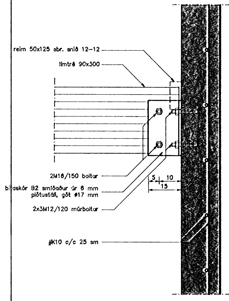
Snið 13-13 Mkv. 1 : 10
