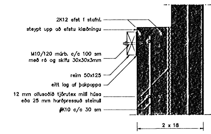
Snið 20-20 Mkv. 1 : 10
