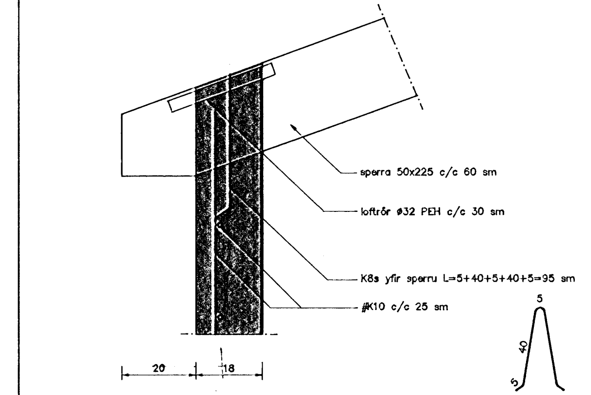
Snið 22-22 Mkv. 1 : 10
