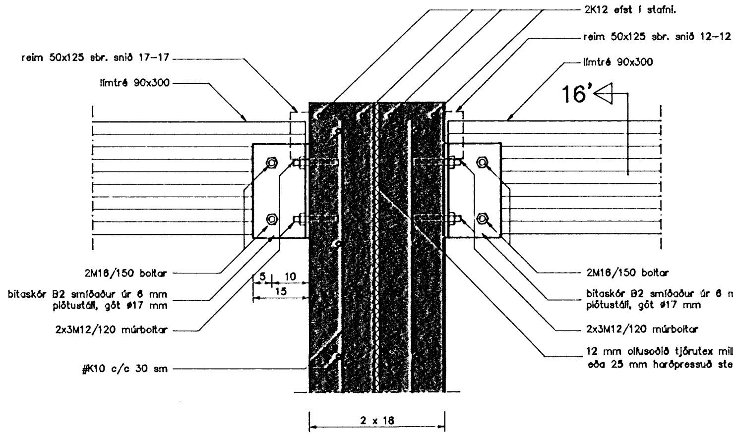
Snið 16-16 Mkv. 1 : 10
