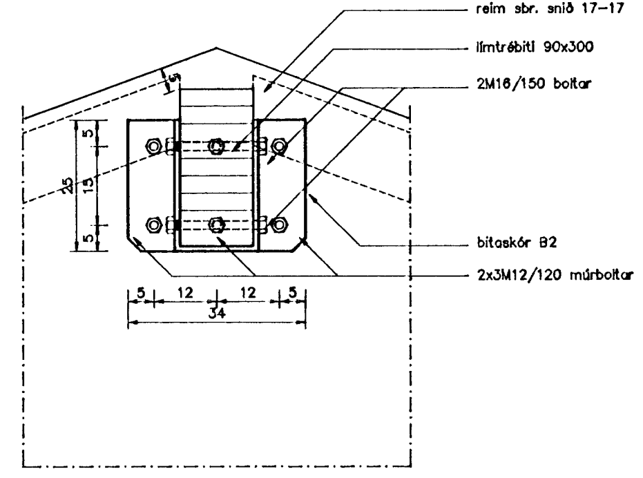
Snið 16'-16' Mkv. 1 : 10
