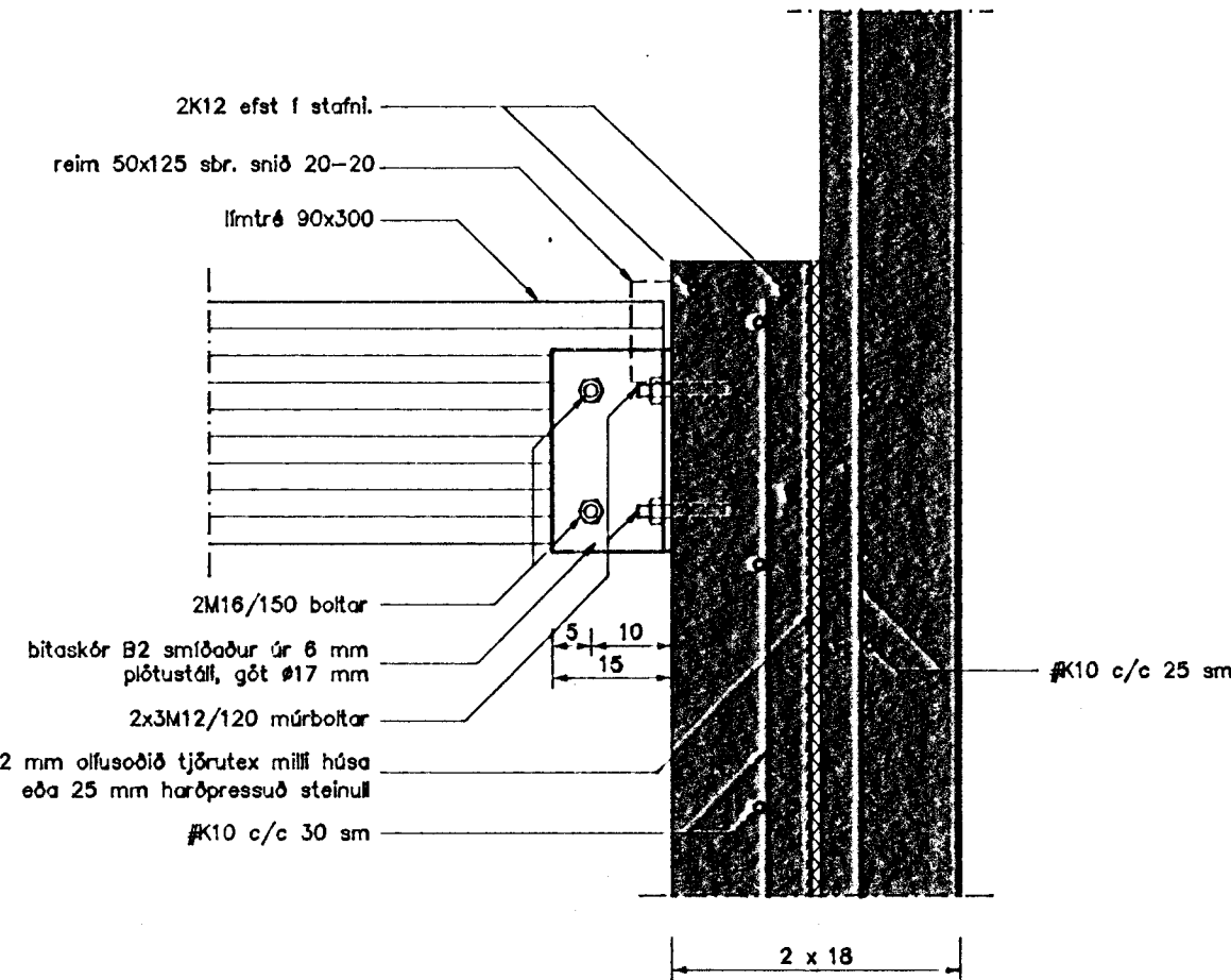
Snið 19-19 Mkv. 1 : 10
