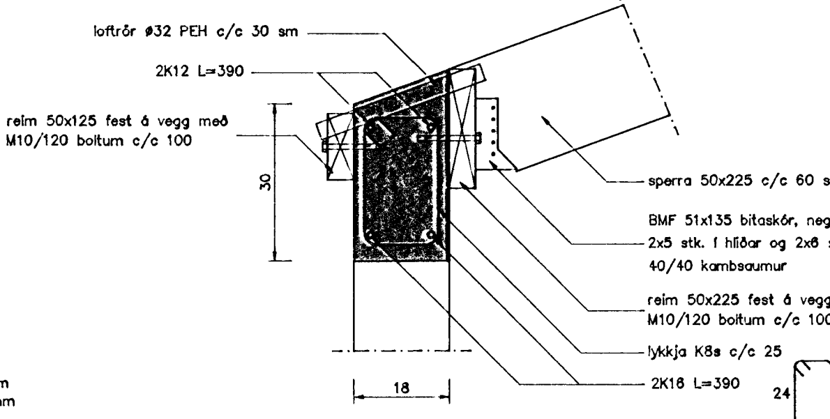
Snið 18-18 Mkv. 1 : 10
