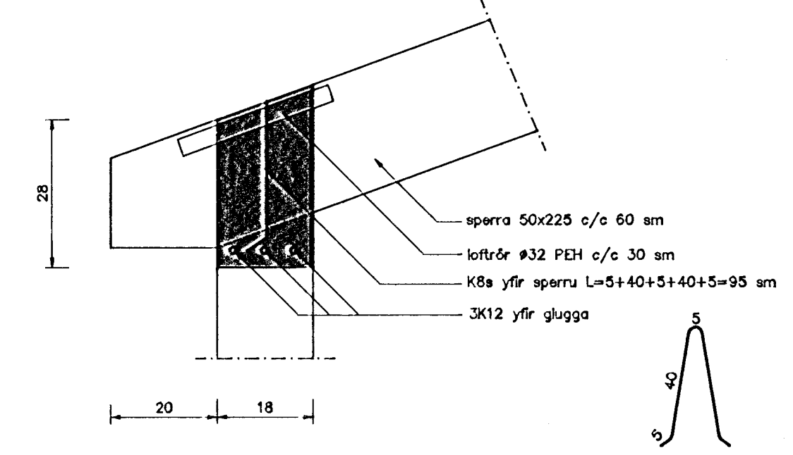
Snið 21-21 Mkv. 1 : 10
