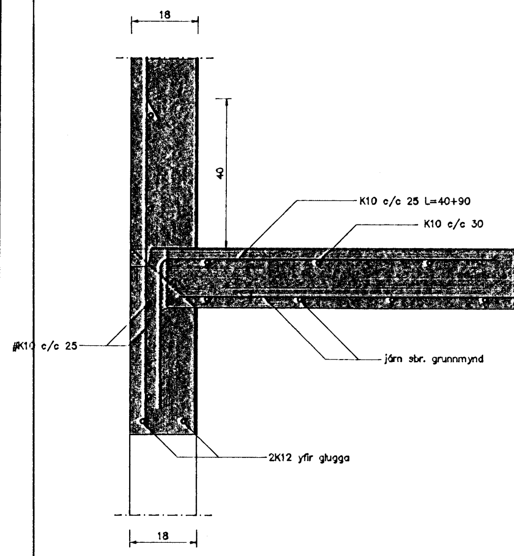
Snið 8-8 Mkv. 1 : 10
