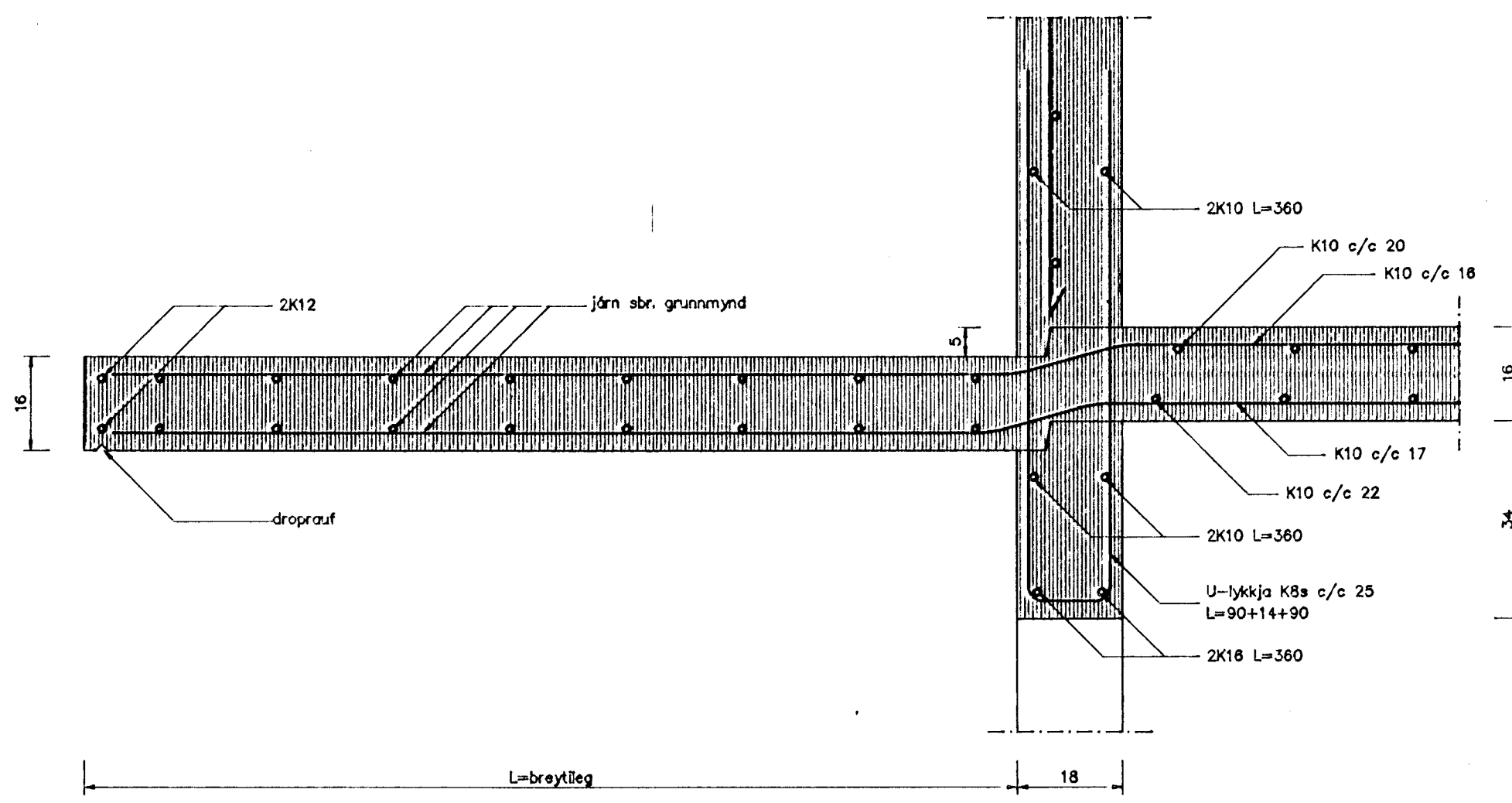
Snið 10-10 Mkv. 1 : 10
