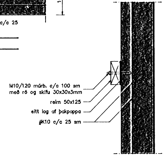
Snið 12-12 Mkv. 1 : 10
