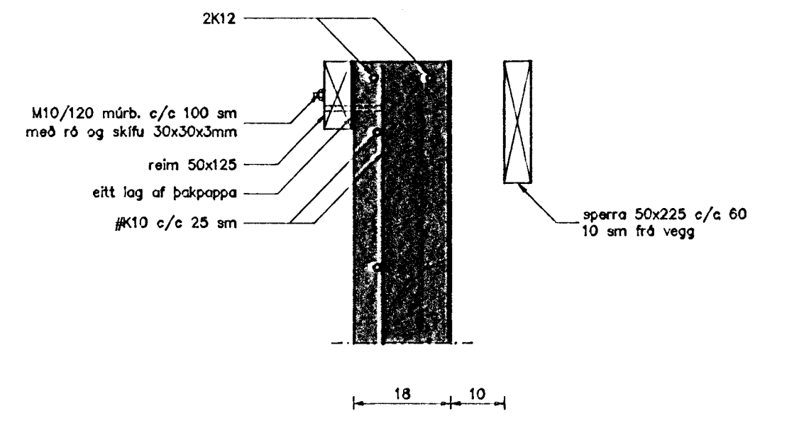
Snið 23-23 Mkv. 1 : 10
