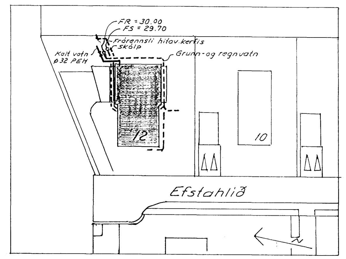
AFSTÖÐUMYND M. 1:500
