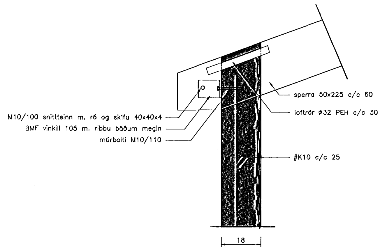
Festing á nýjum sperrum Mkv. 1:10
