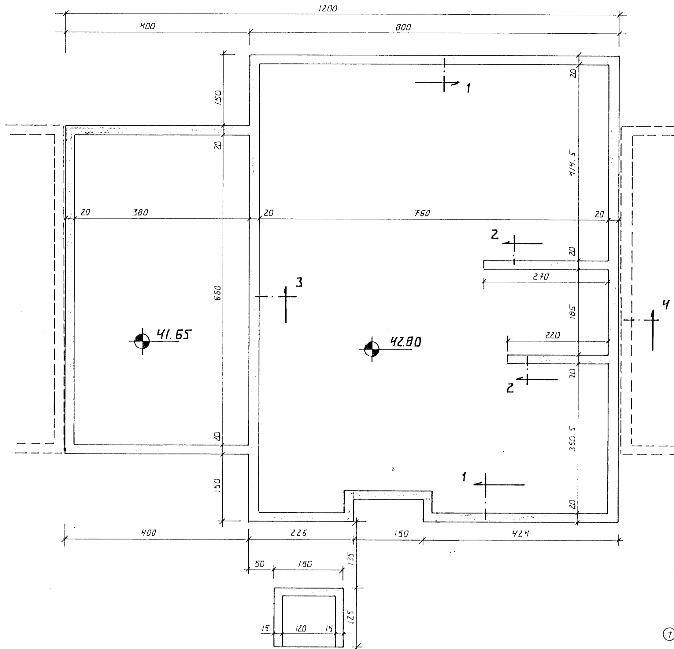
GRUNNMÝND, 1:50
