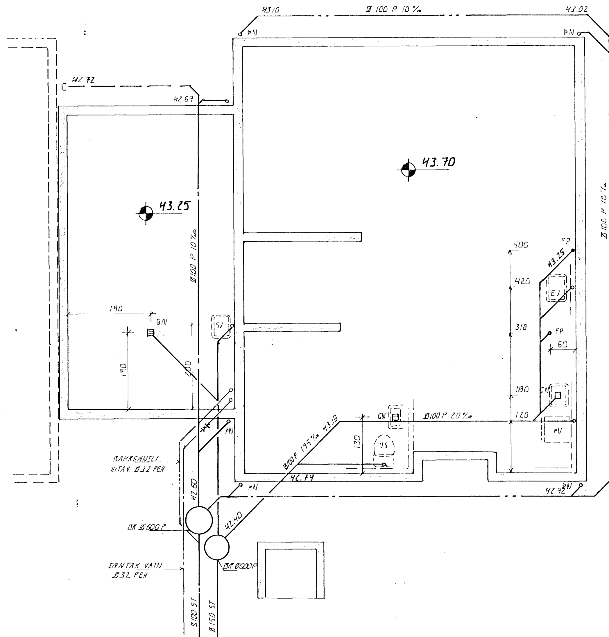
GRUNNMÝND, 1:50
