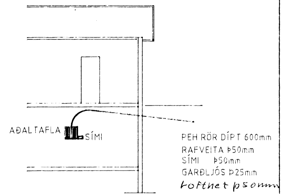
SNID A-A
