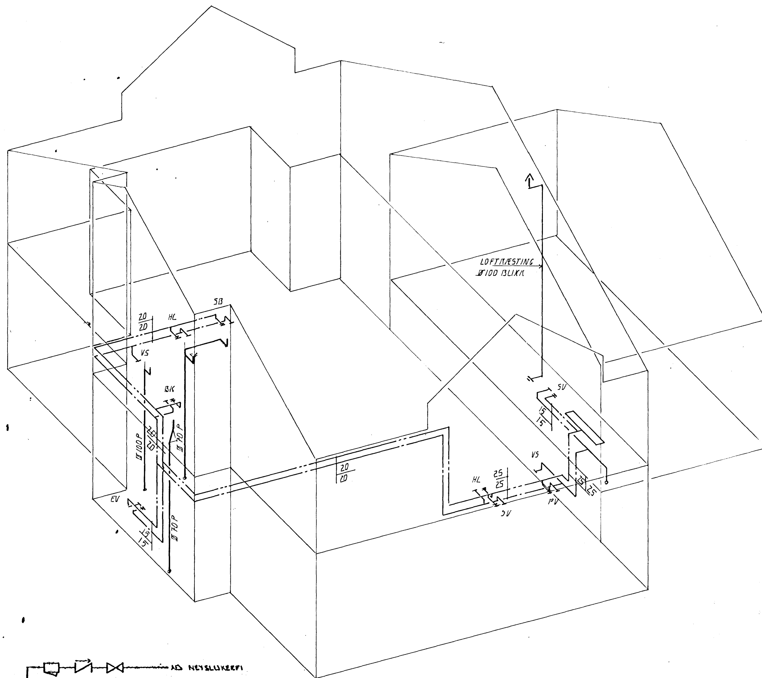
VATNS - OG FRÁRENNSLISLAGNIR RÚMMYND, 1:50
