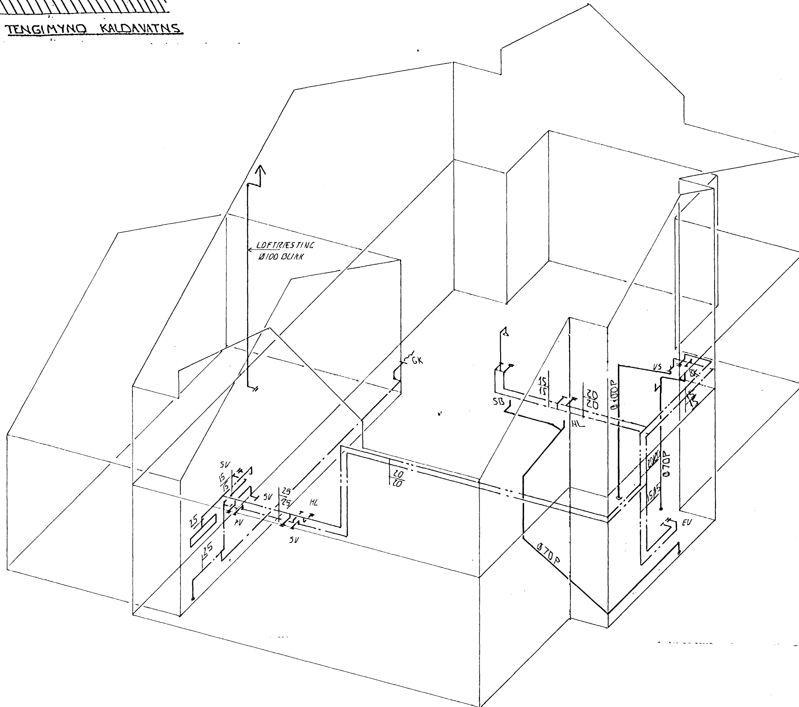
VATNS. OG FRÆRENNSLISLAGNIR. RÚMMYND. 1:50
