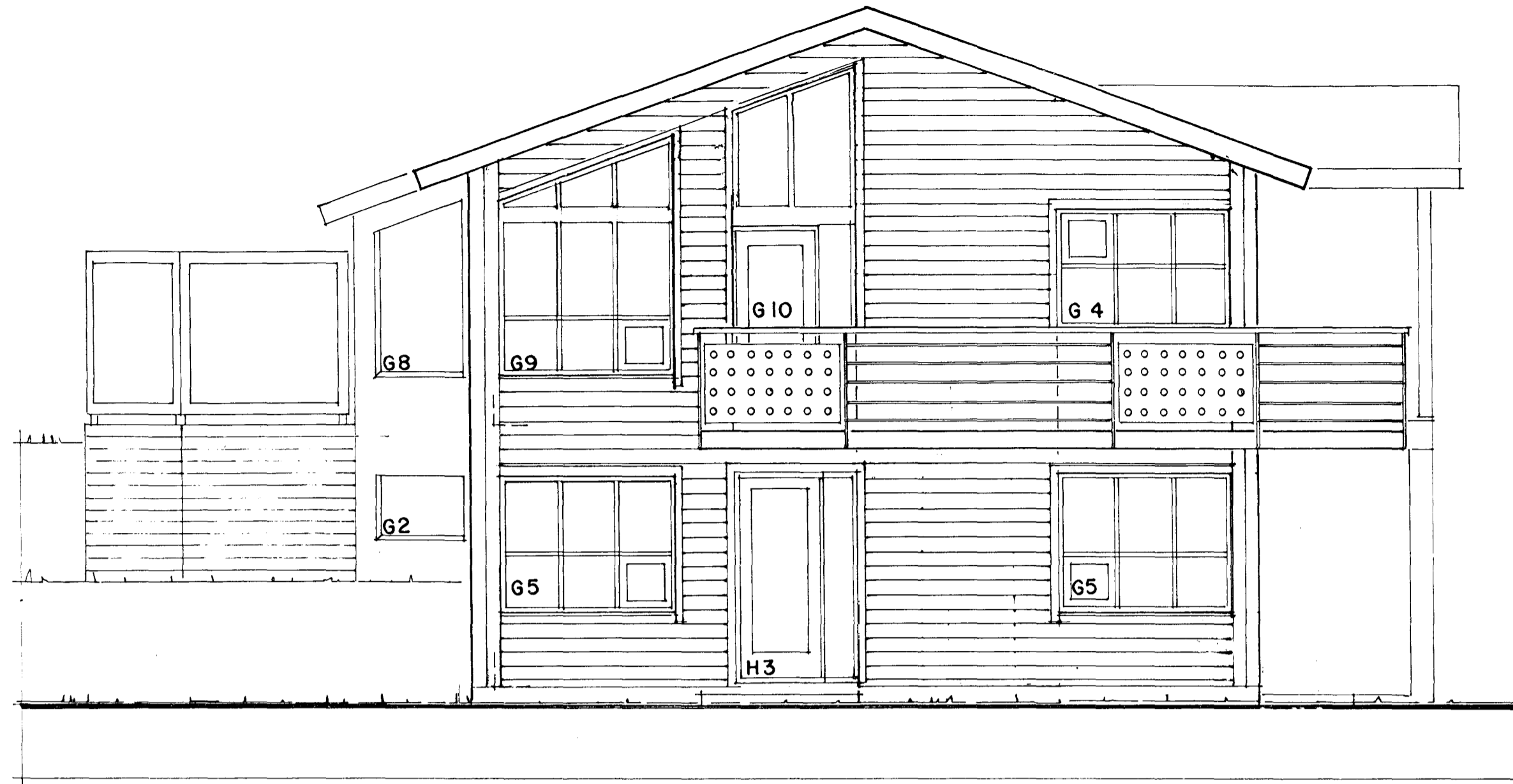
ÚTLIT AUSTUR 1:50
