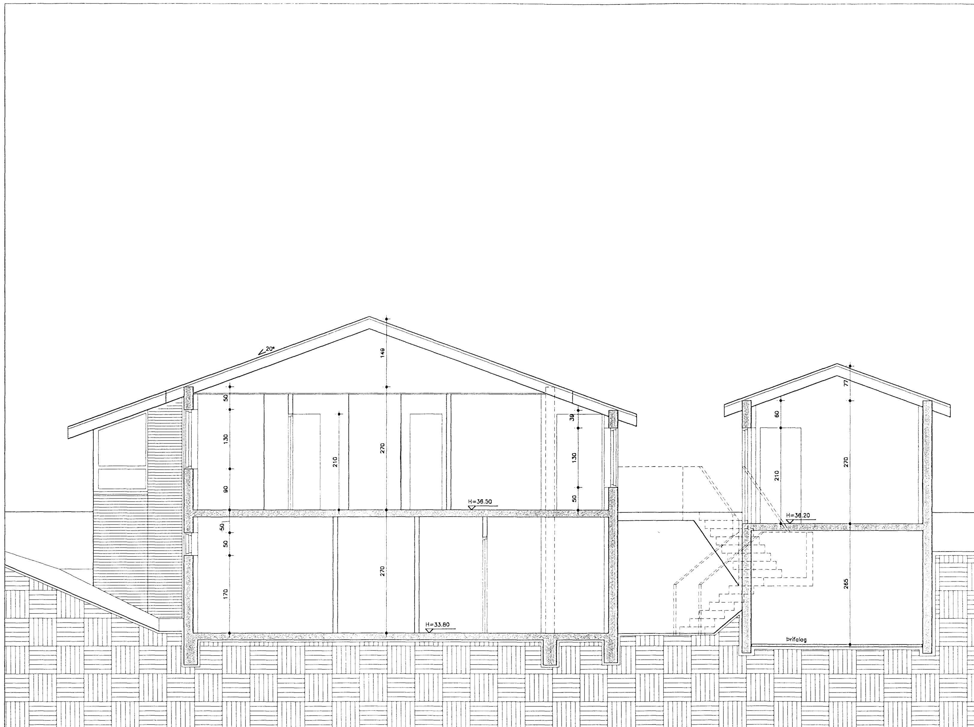
SNID A-A
