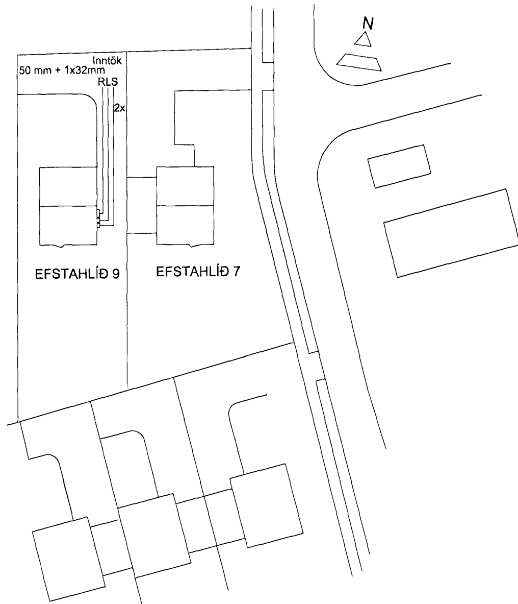
AFSTÖÐUMYND - 1:500
