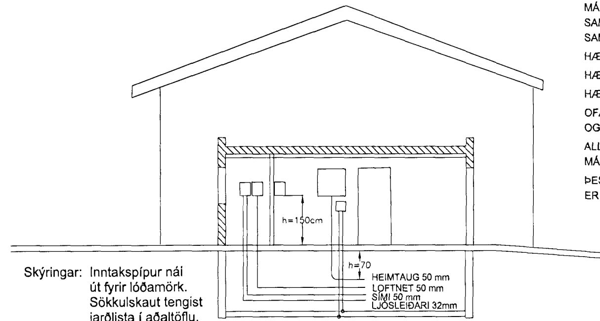
SNIÐMYND - 1:100
