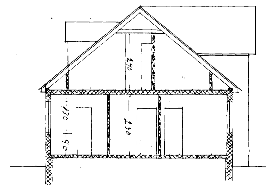
Þverskurður
