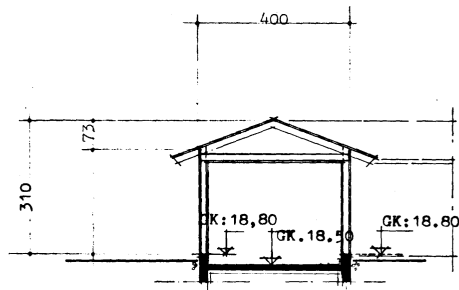
ÞVERSNIÐ A - A
