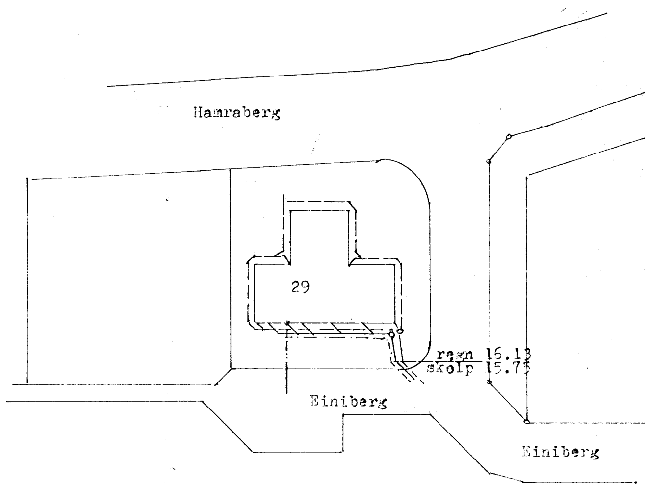
Aðstöðuneynd M=1:500
