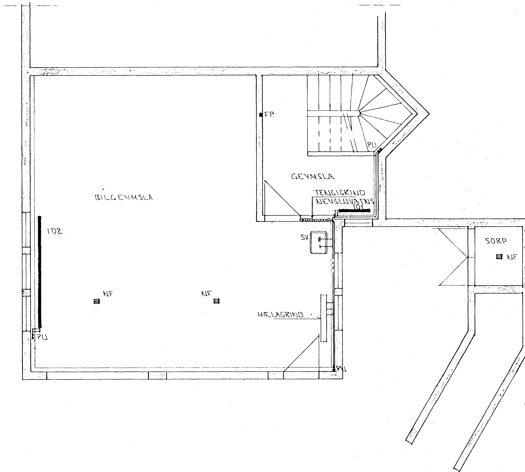
GRUNNMYND 1 HÆÐ 1:50
