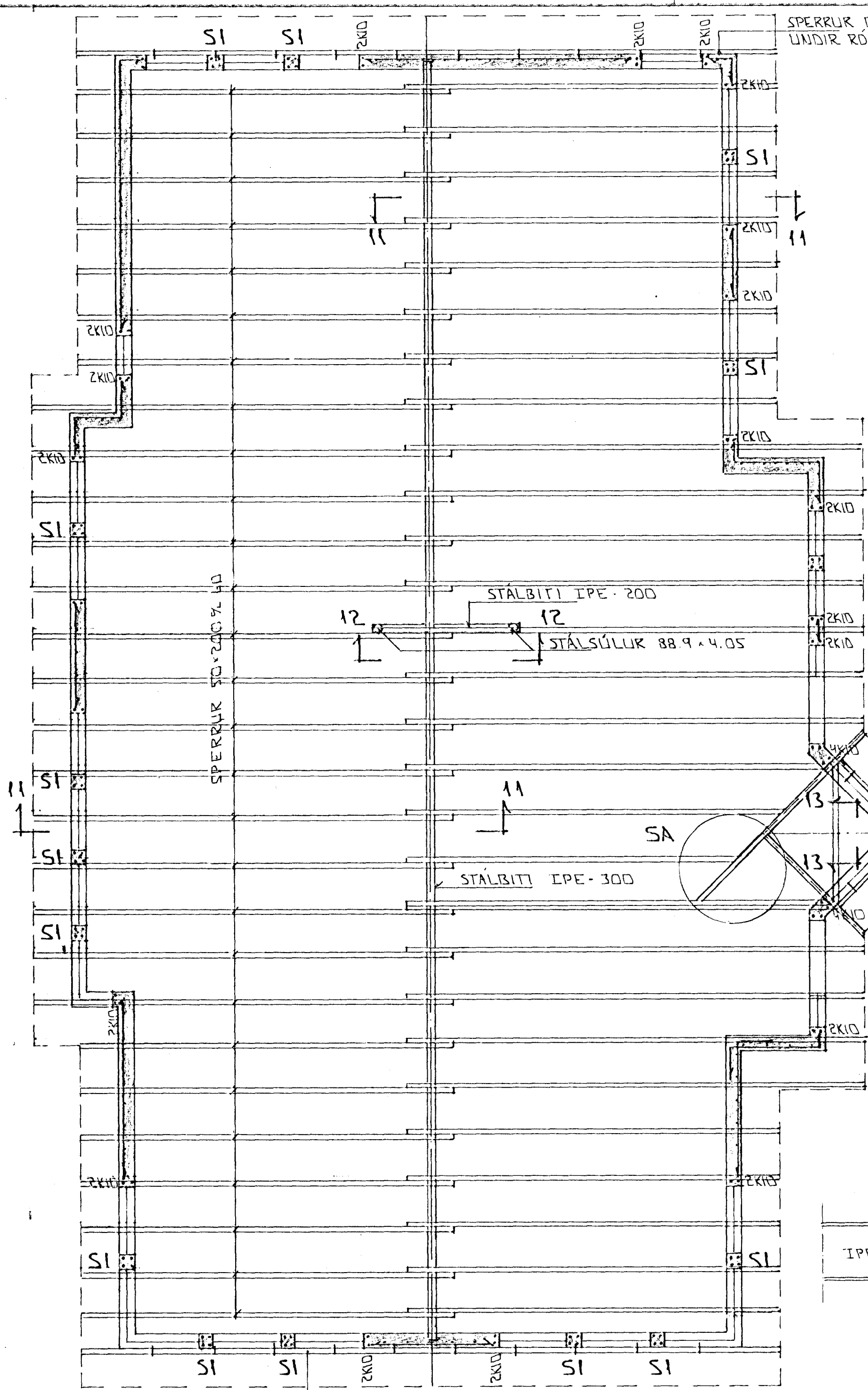
GRUNNMÝND 1:50
