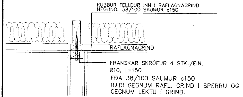
SNÍÐ VIÐ SPERRU Mkv. 1:10
