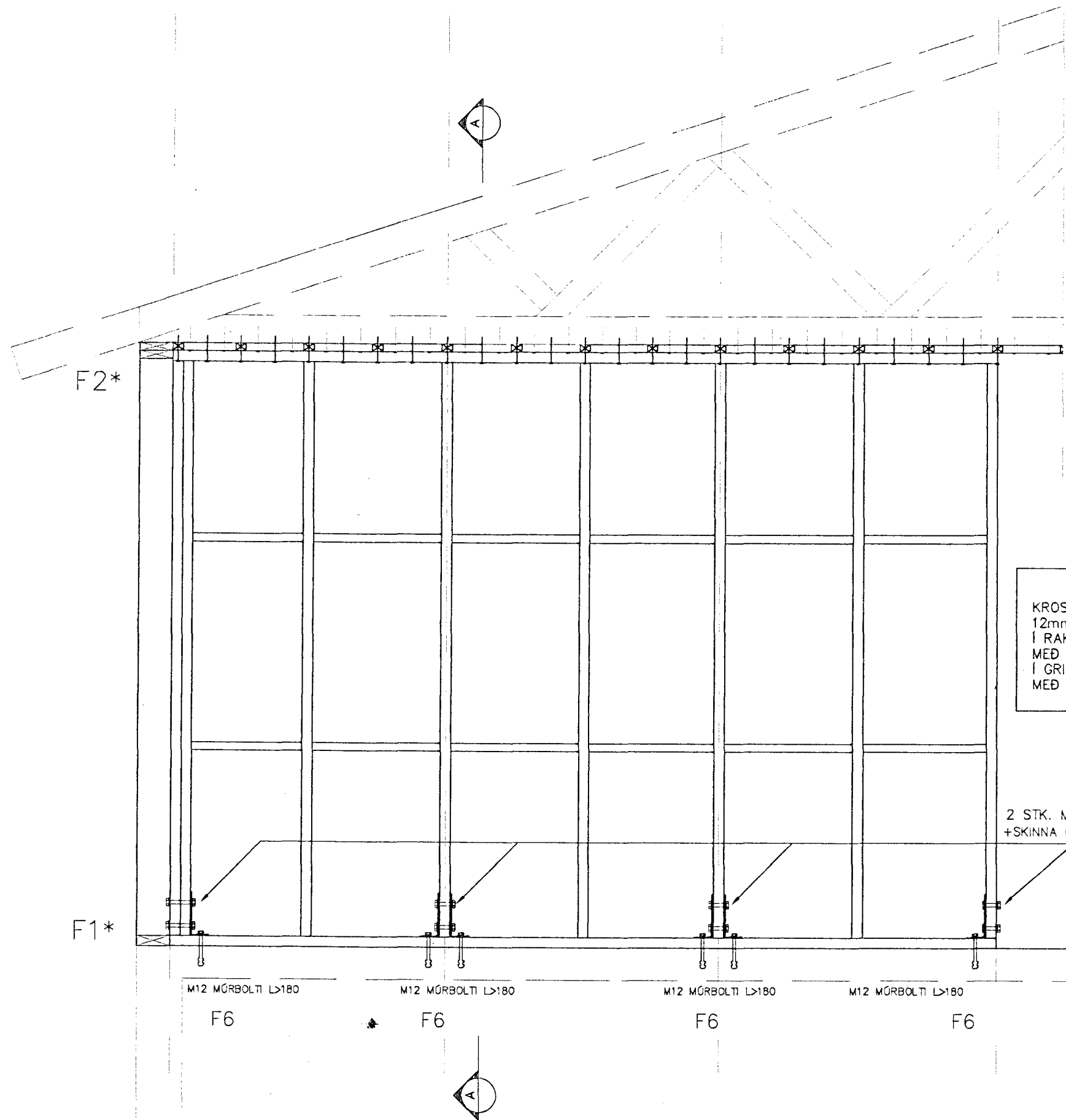
STÍFINGARVEGGUR Mkv. 1:20
