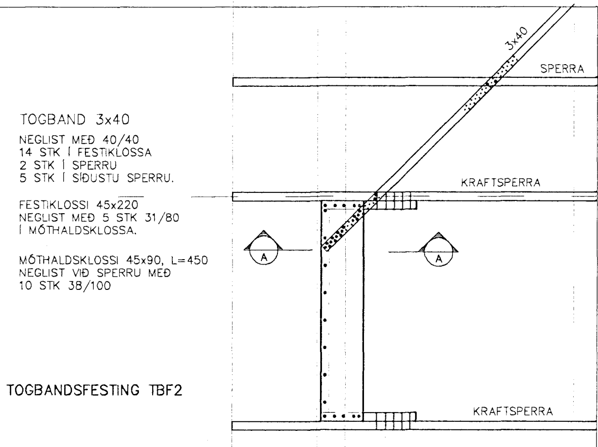
FESTING TOGBANDA Í ÞAKI 1:20
