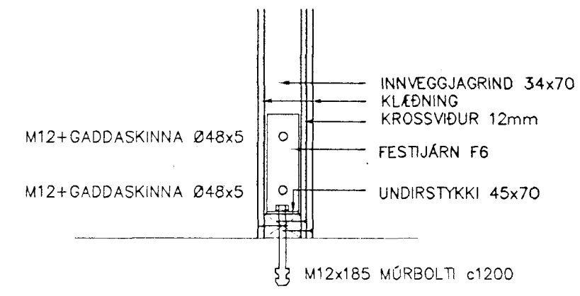
SNÍÐ A-A VIÐ GÓLF Mkv. 1:10
