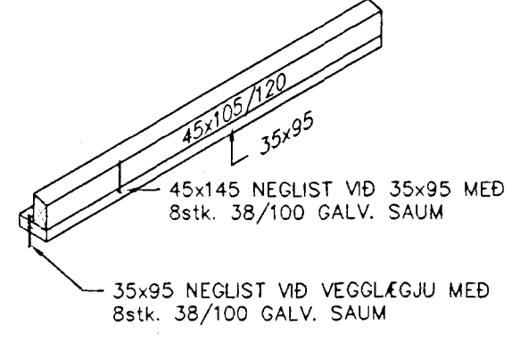
SPERRUKLOSSI 1:20
