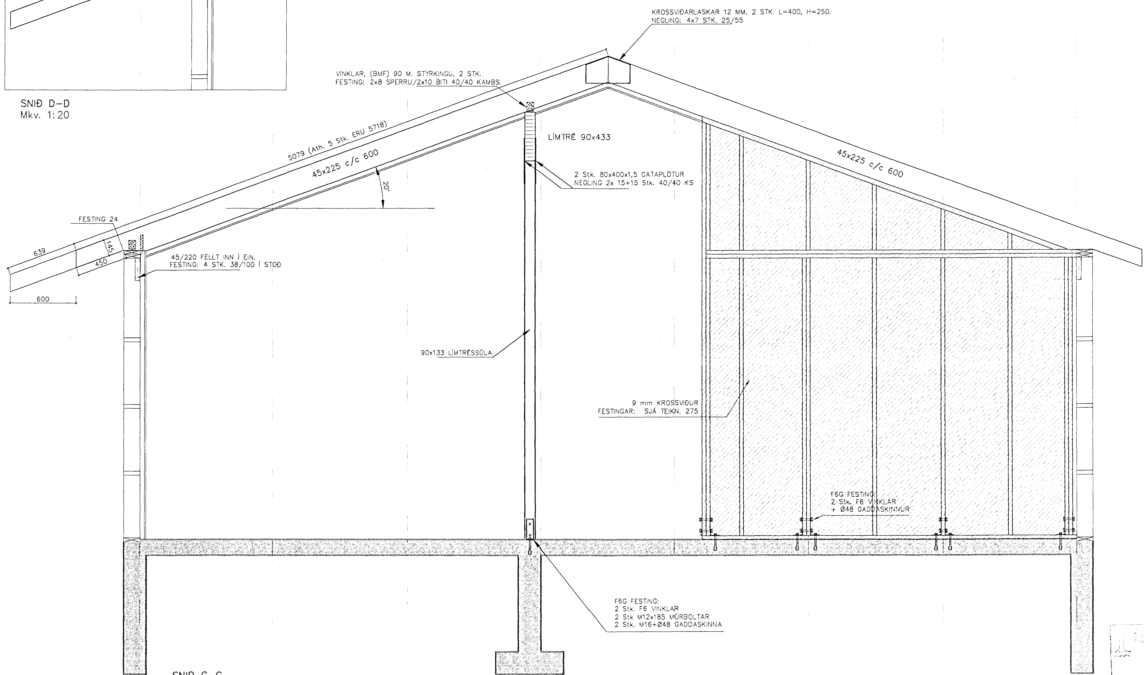
SNID C-C Mkv. 1:20
