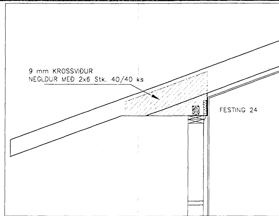
SNID D-D Mkv. 1:20
