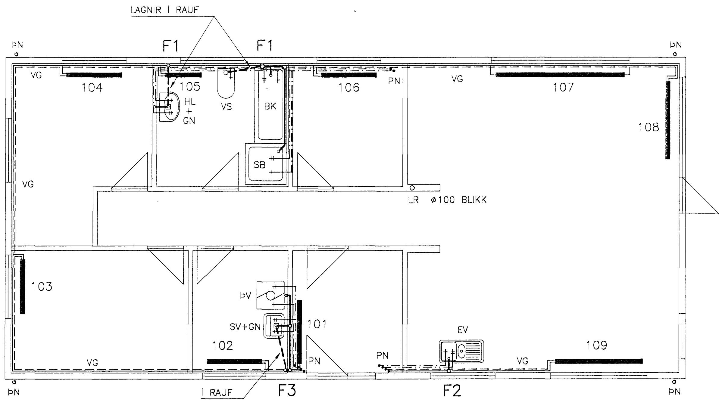
GRUNNMYND EFRI HÆÐAR 1:50
