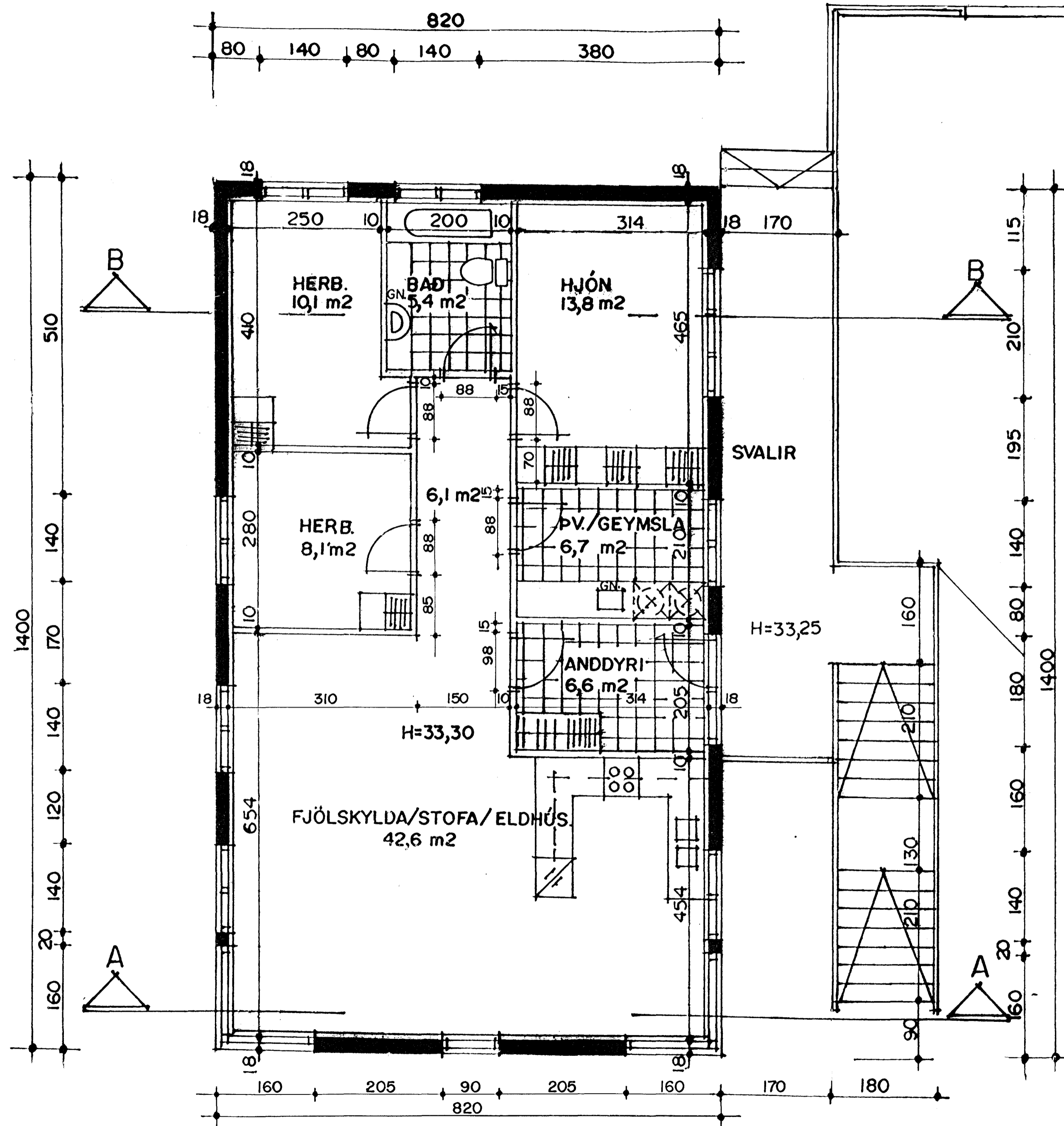
GRUNNMYND 2 HÆÐ MKV. 1:50.
