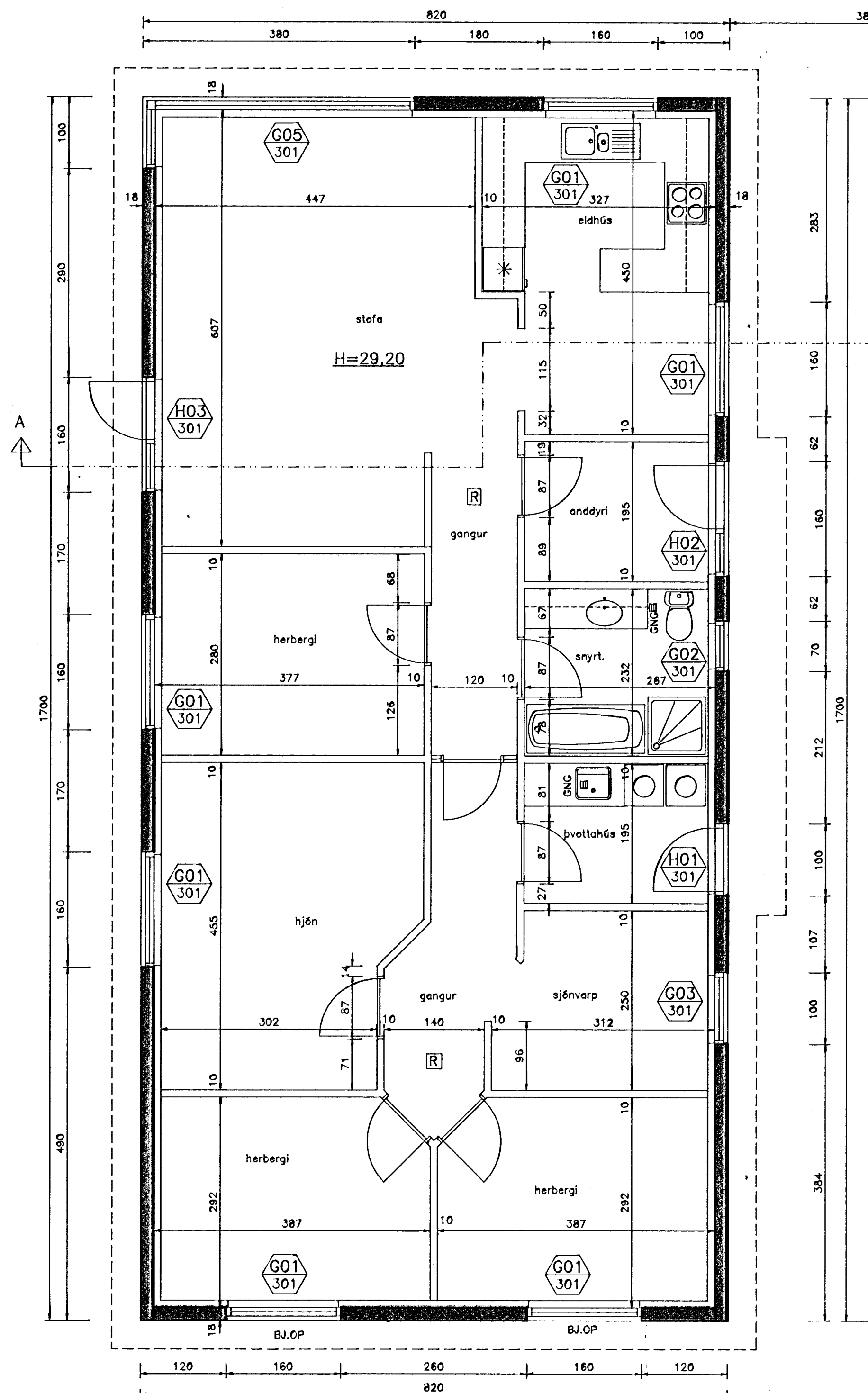
MÁLTEIKNING GRUNNMYND MKV. 1:50
