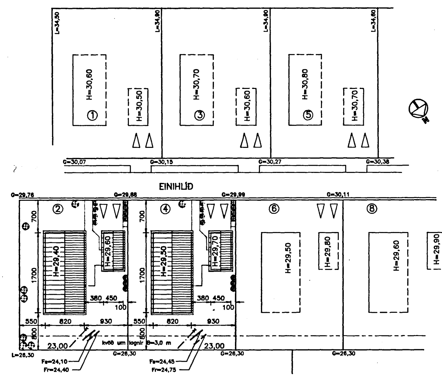
AFSTÖÐUMYND mkv. 1:500
