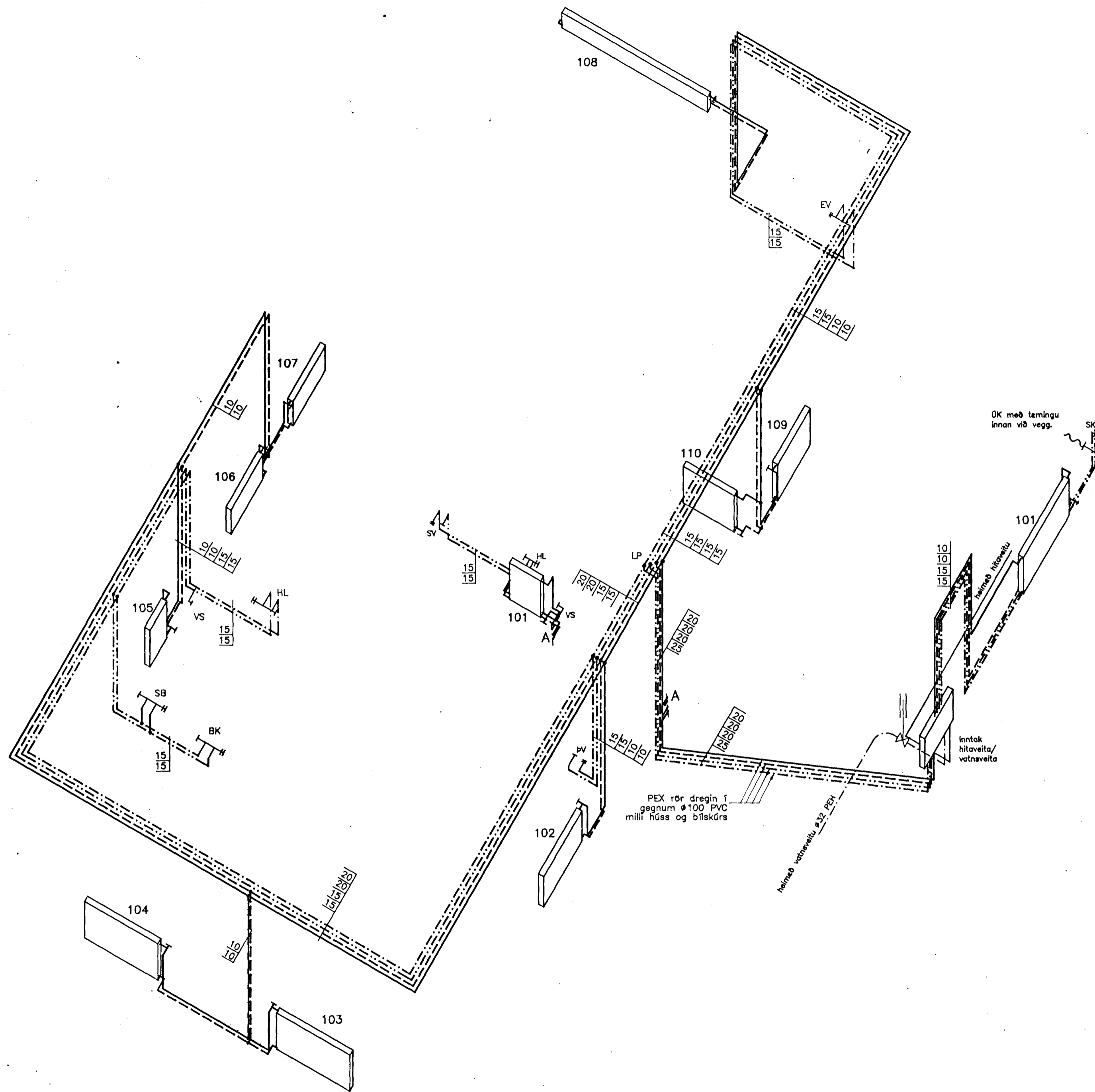
Rúmmynd neysluvatns- og hitalagna mkv. 1:50
