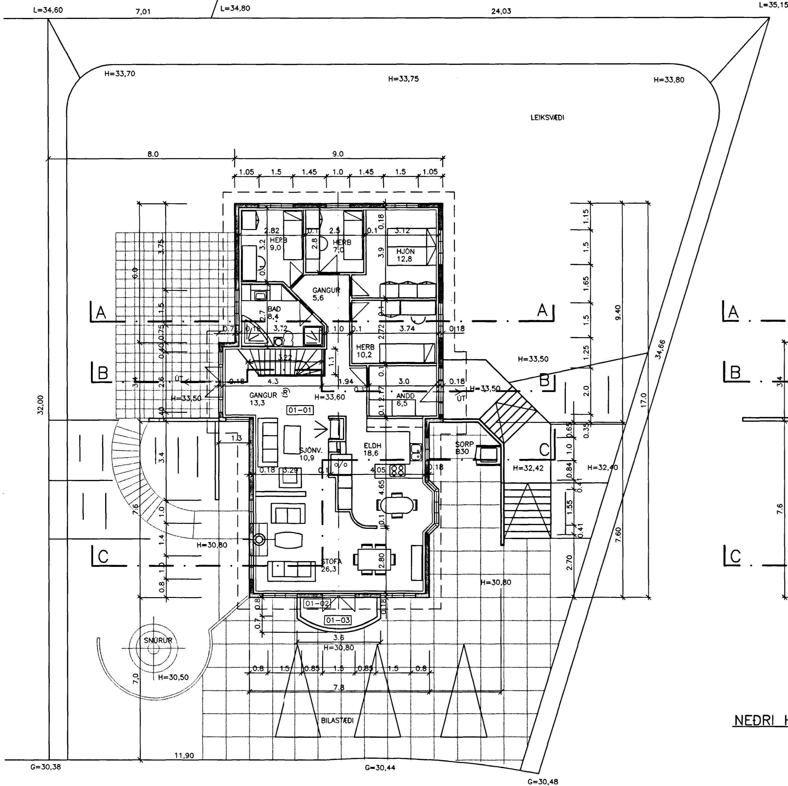
EFRI HÆÐ, GRUNNMYND
