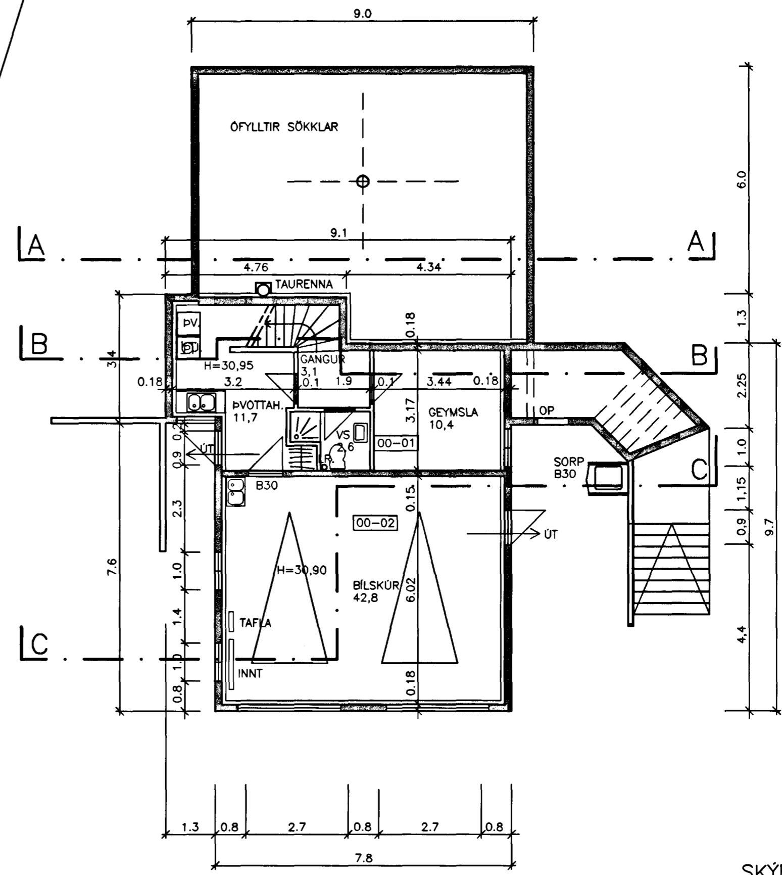
NEDRI HÆÐ, GRUNNMYND
