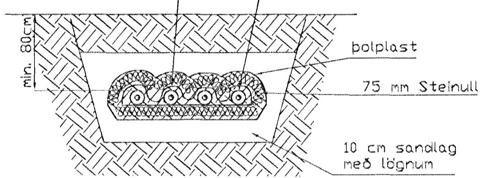
Lagnir í jörð, Sníð 1, 1:20
