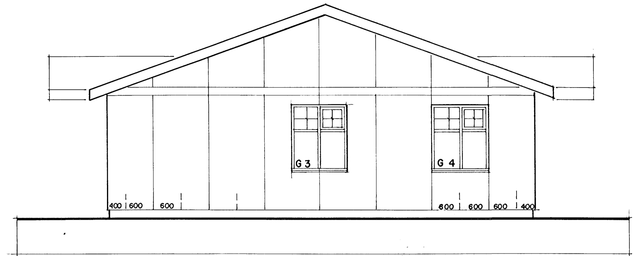
ÚTLIT SUÐUR 1:50
