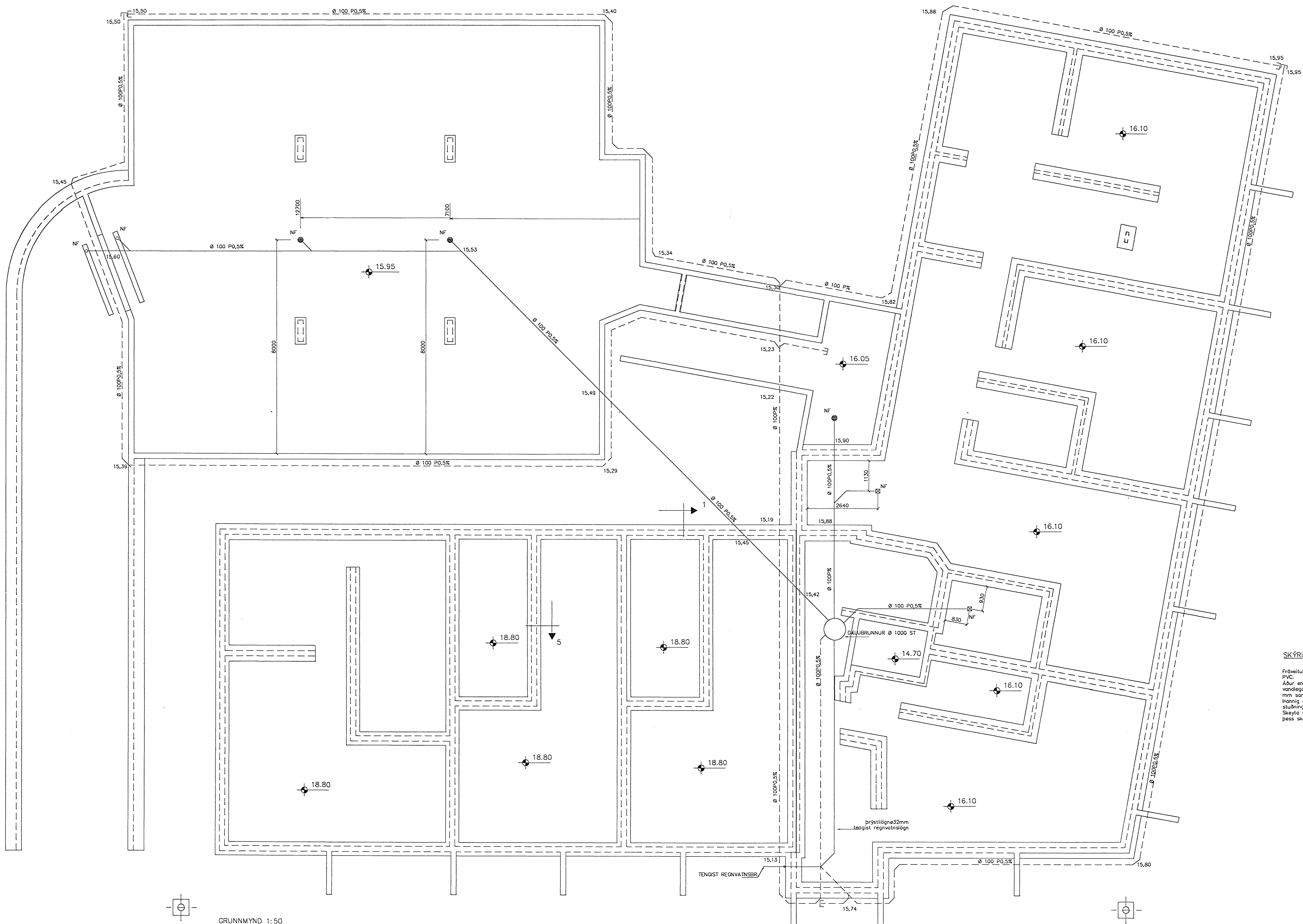
GRUNNMYND 1:50
