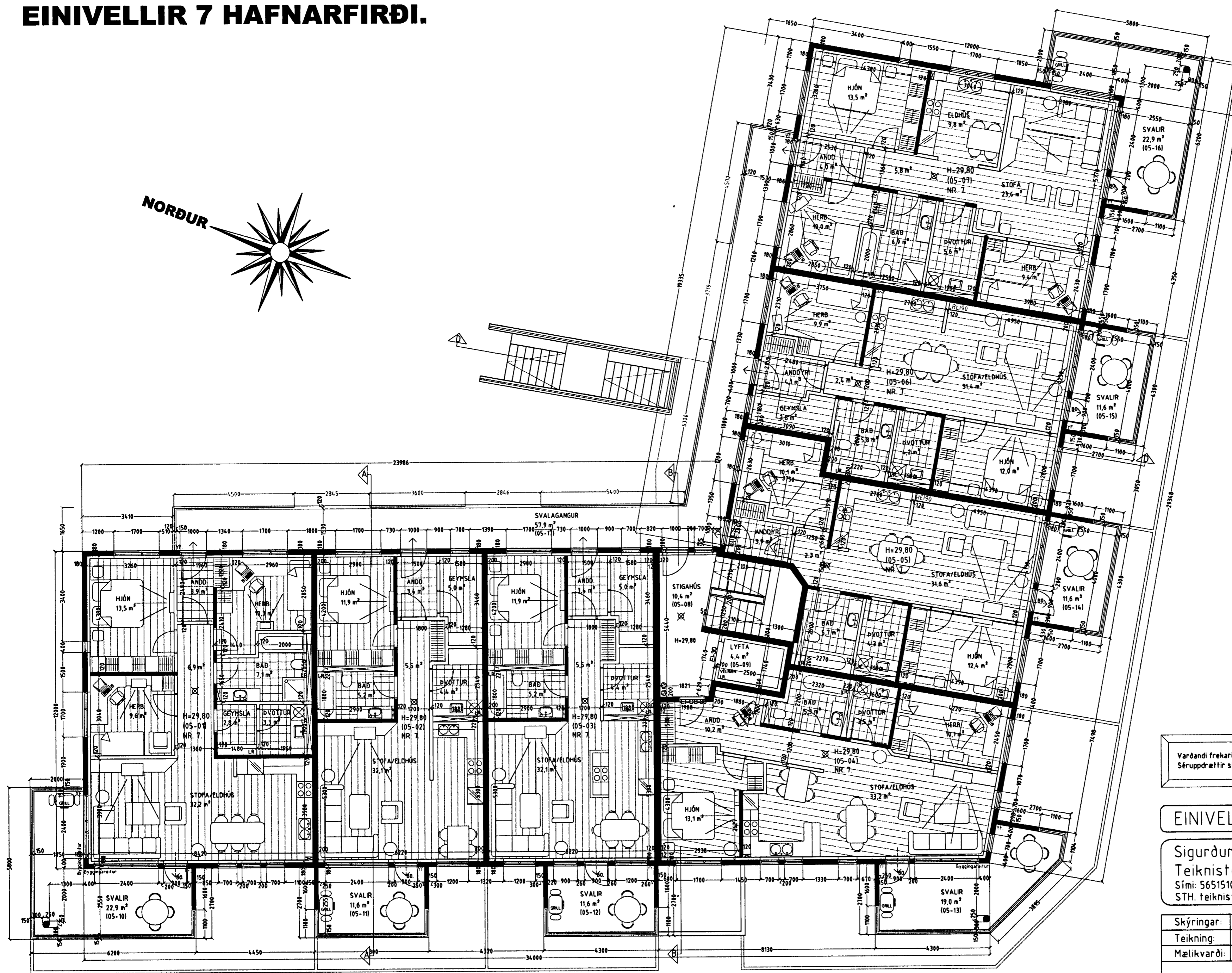
GRUNNMYND 5. HÆÐ MKV. 1:100.
