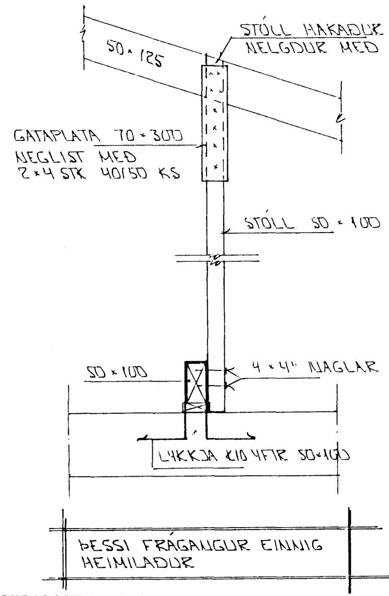
SNID 6 - 1:10
