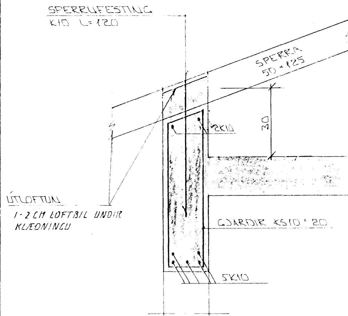
SNID 6 - 1:10
