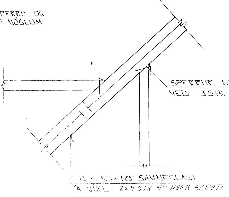
SERMYND A - 1:10
