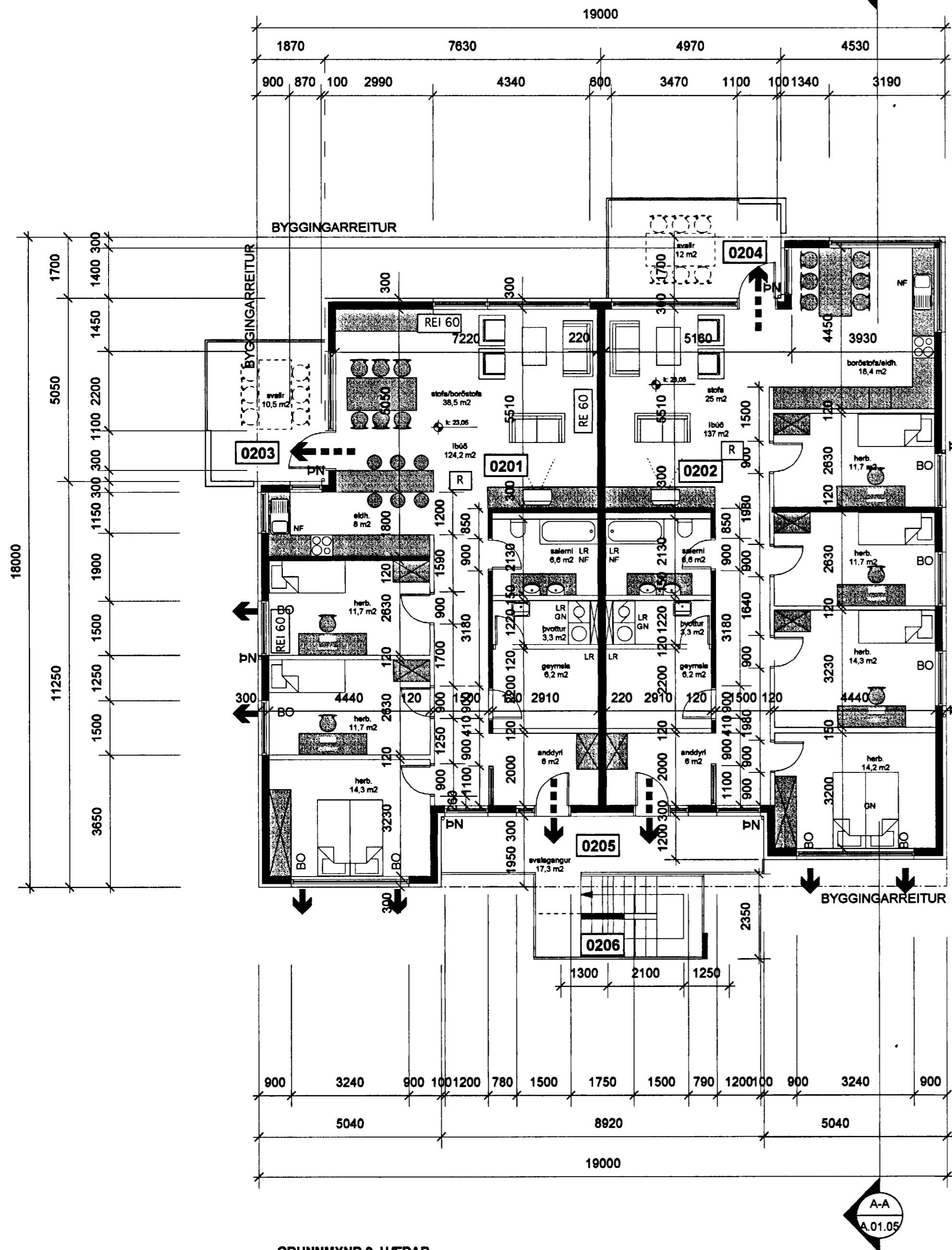
GRUNNMYND 2. HÆÐAR mkv. 1:100
