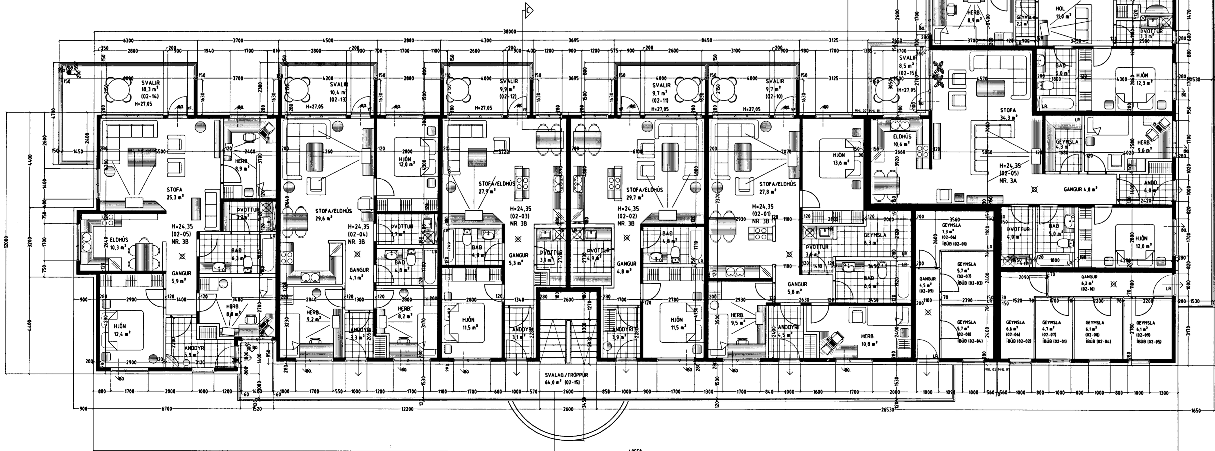
GRUNNMYND 2. HÆÐ MKV. 1:100.
