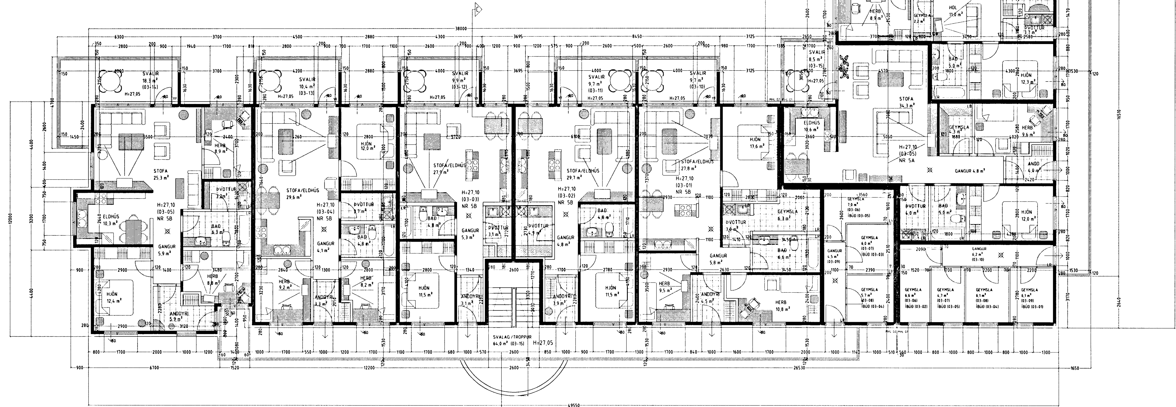
GRUNNMYND 3. HÆÐ MKV. 1:100.
