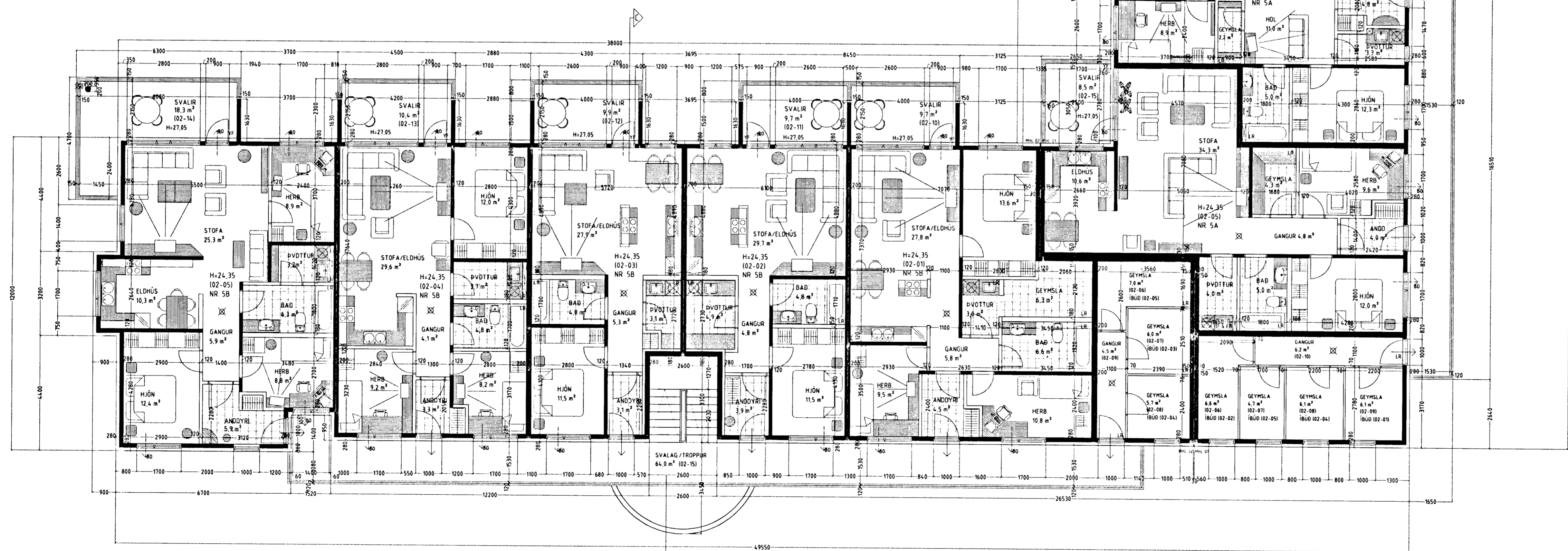
GRUNNMYND 2. HÆÐ MKV. 1:100.
