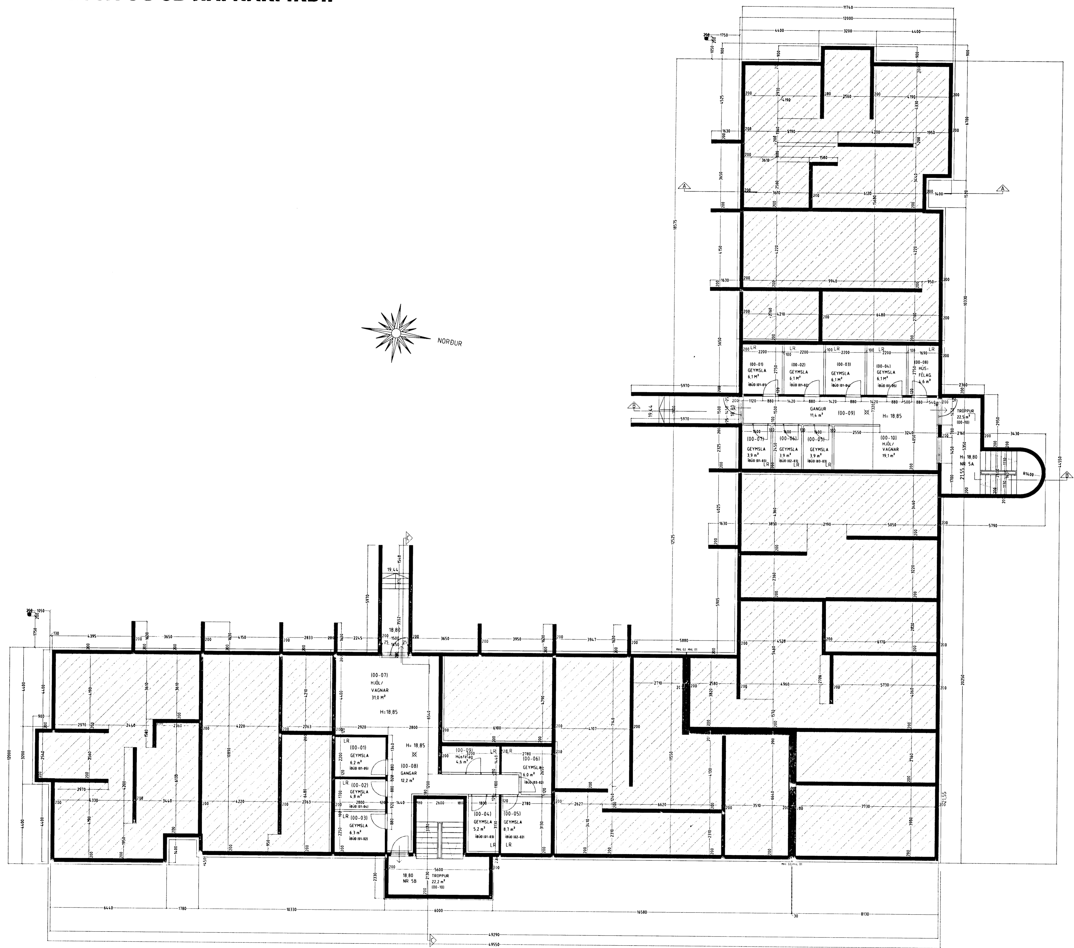
GRUNNMYND KJALLARA MKV. 1:100.
