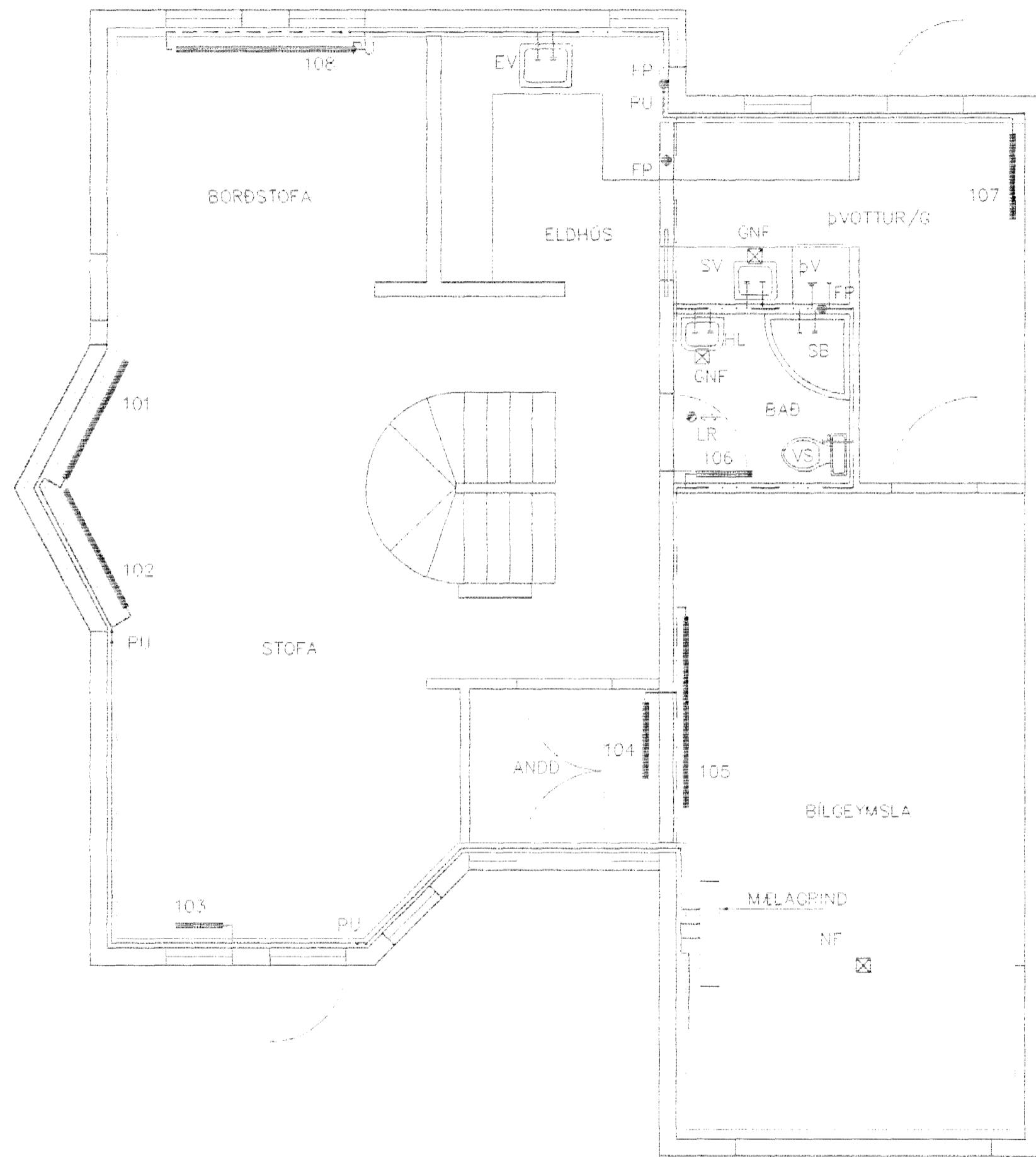
GRUNNMYND 1 HÆÐ 1:50
