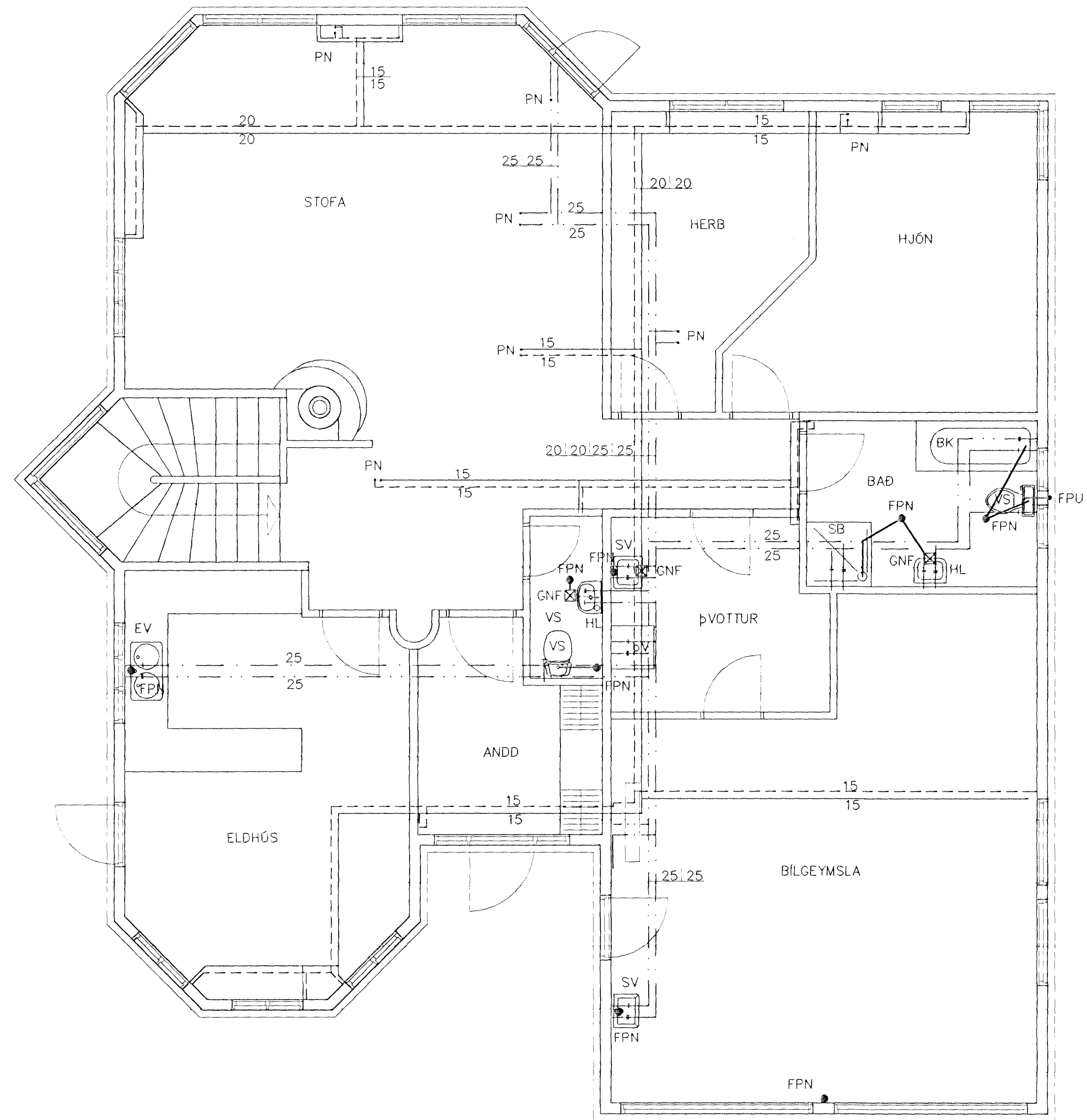
GRUNNMYND 2 HÆÐAR 1:50
