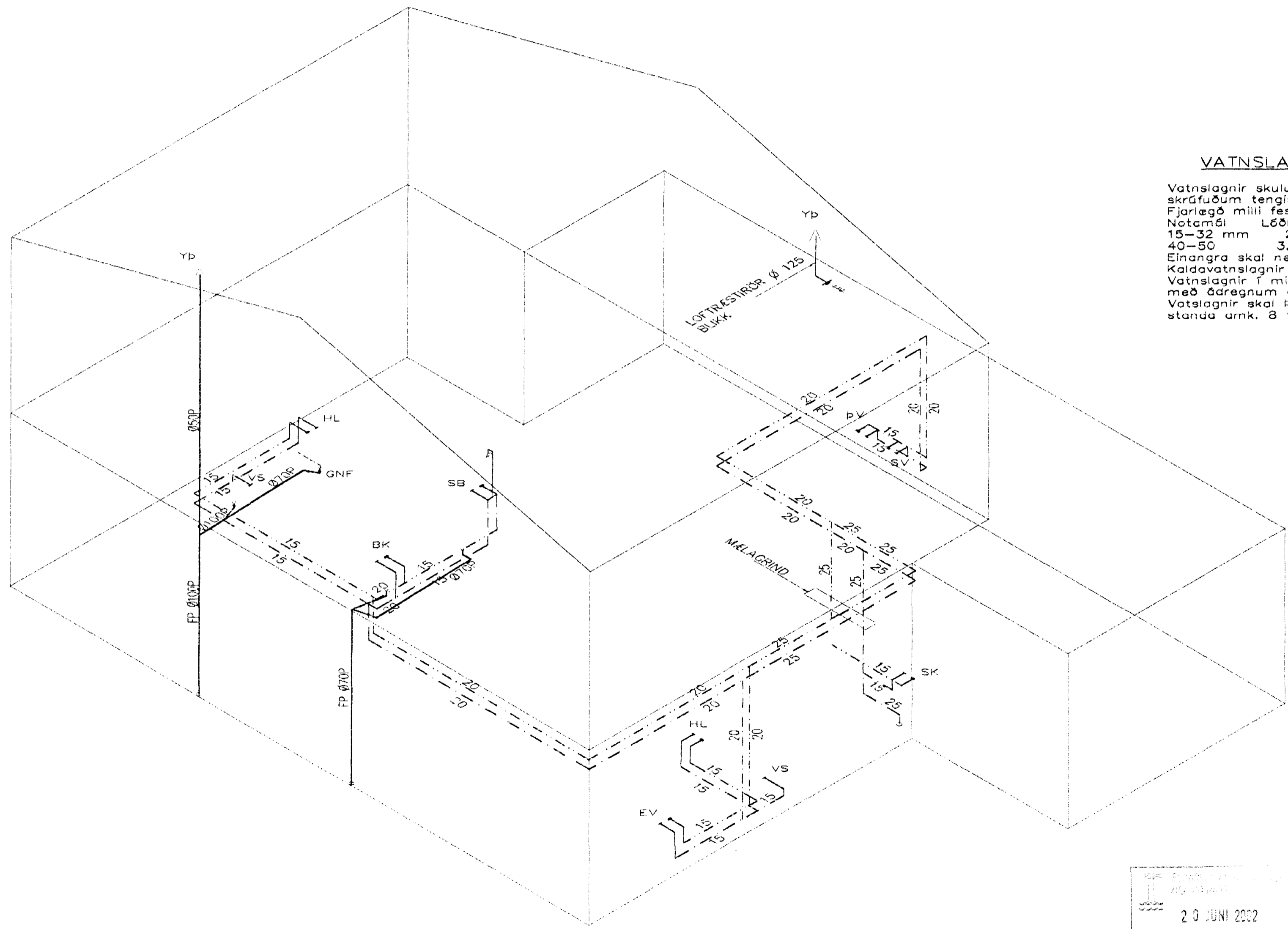
RÚMMYND VATNS OG LOFTRÆSTILAGNA 1:50
