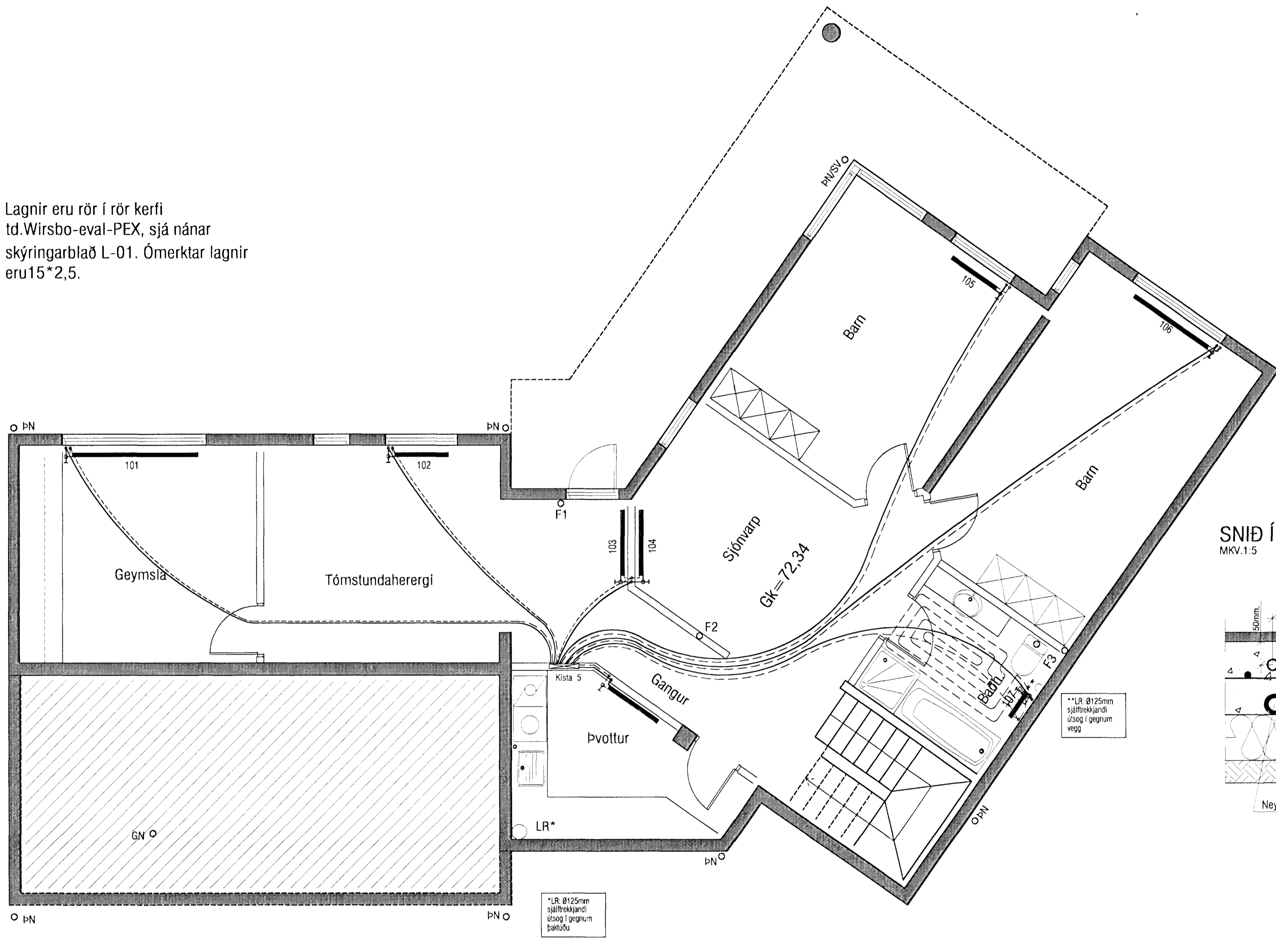
GRUNNMYND 1. HÆÐAR m.k.v 1:50
