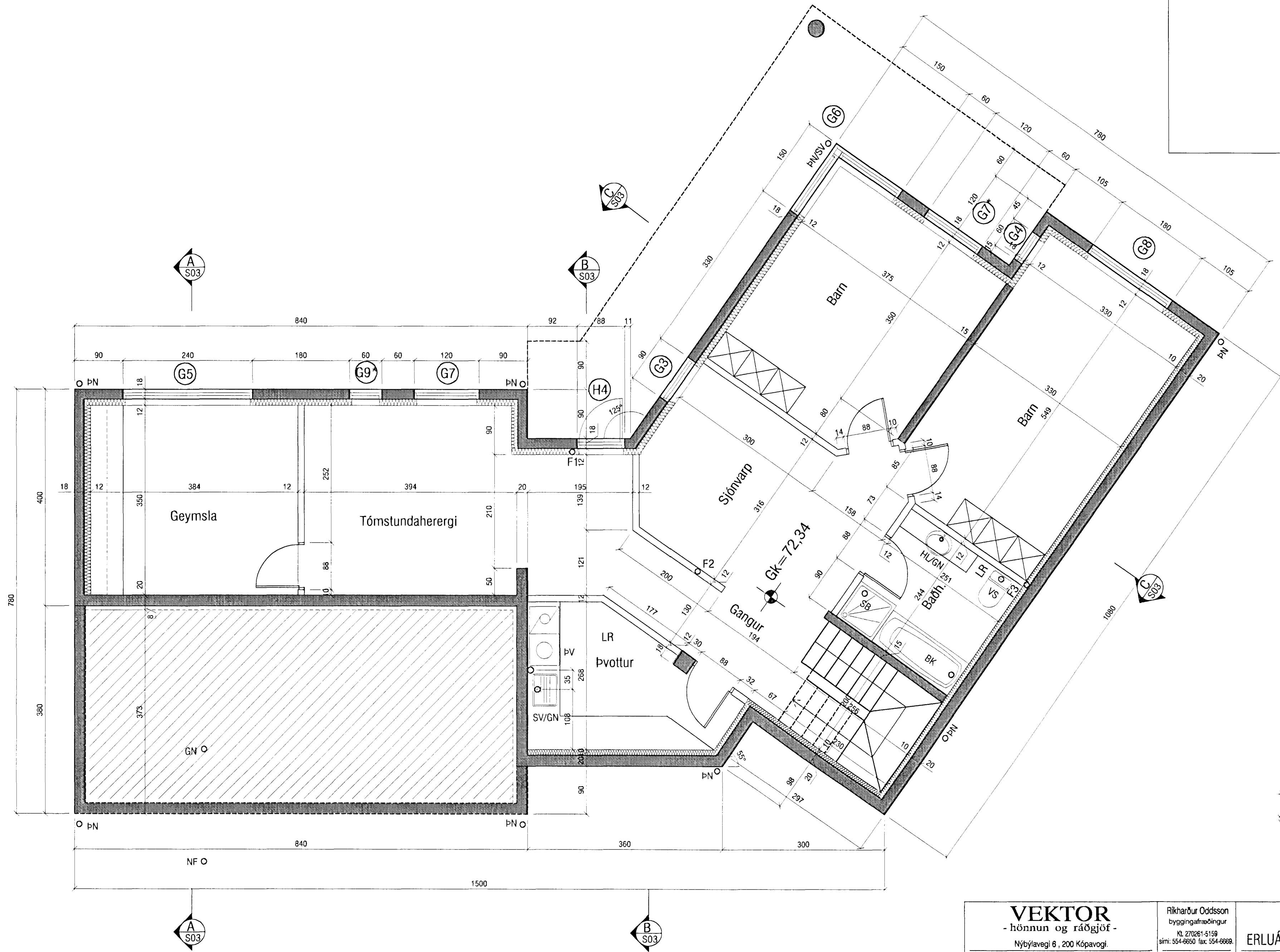
GRUNNMYND 1. HÆÐAR m.k.v 1:50
