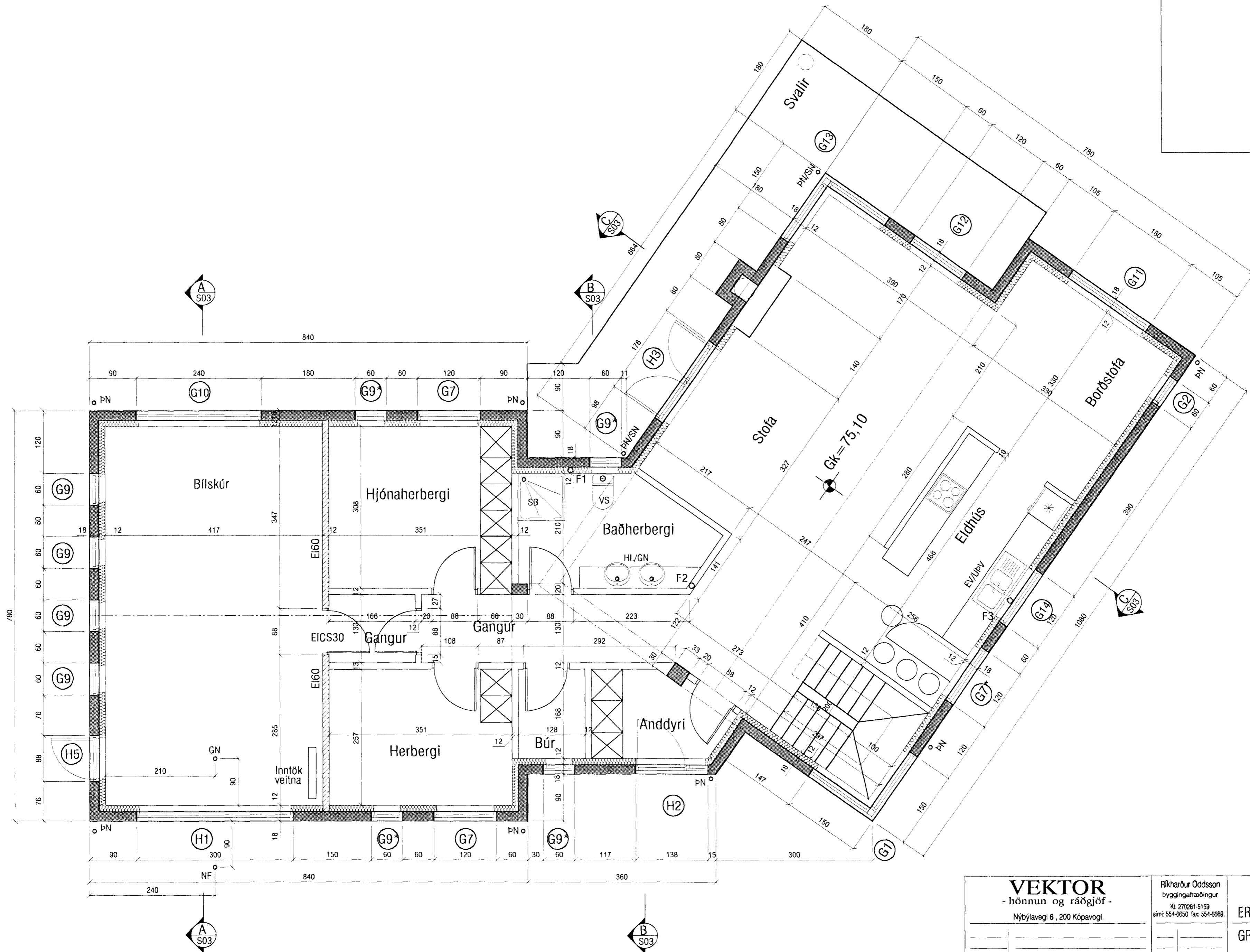
GRUNNMYND 2. HÆÐAR m.k.v 1:100
