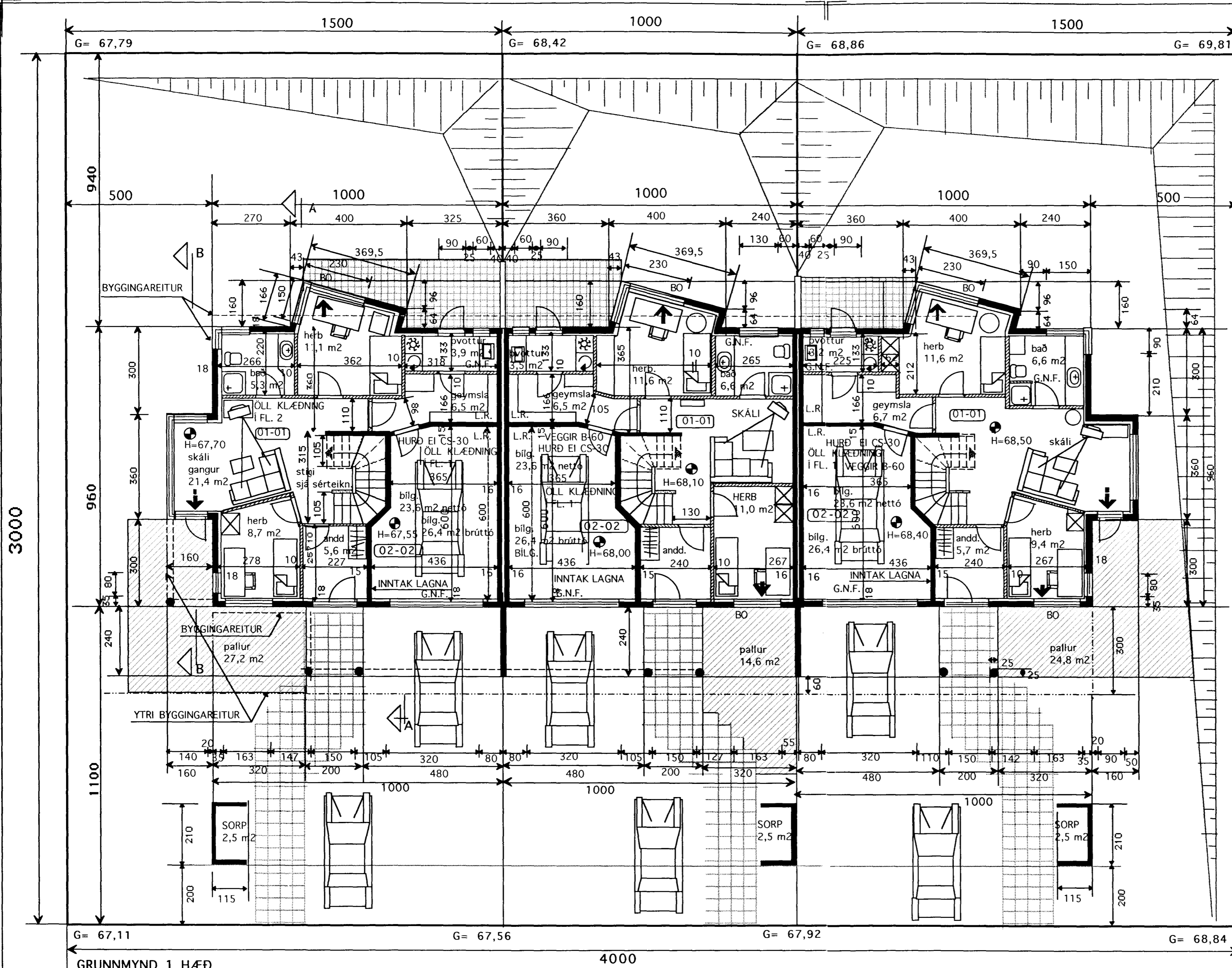
GRUNNMYND 1 HÆÐ NÁNARI MÁLSETNING SJÁ TEKN. V-1 1 :50
