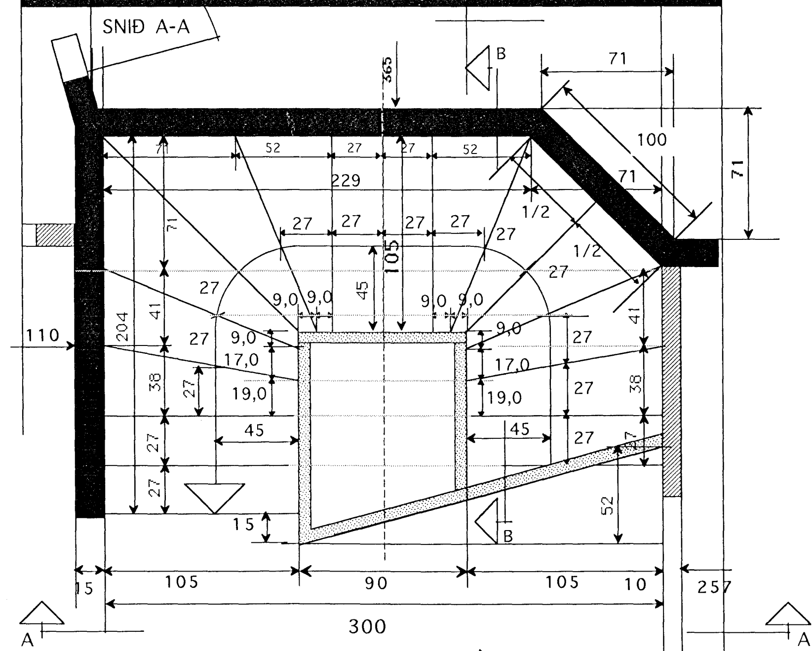
GRUNNMYND 1:20
