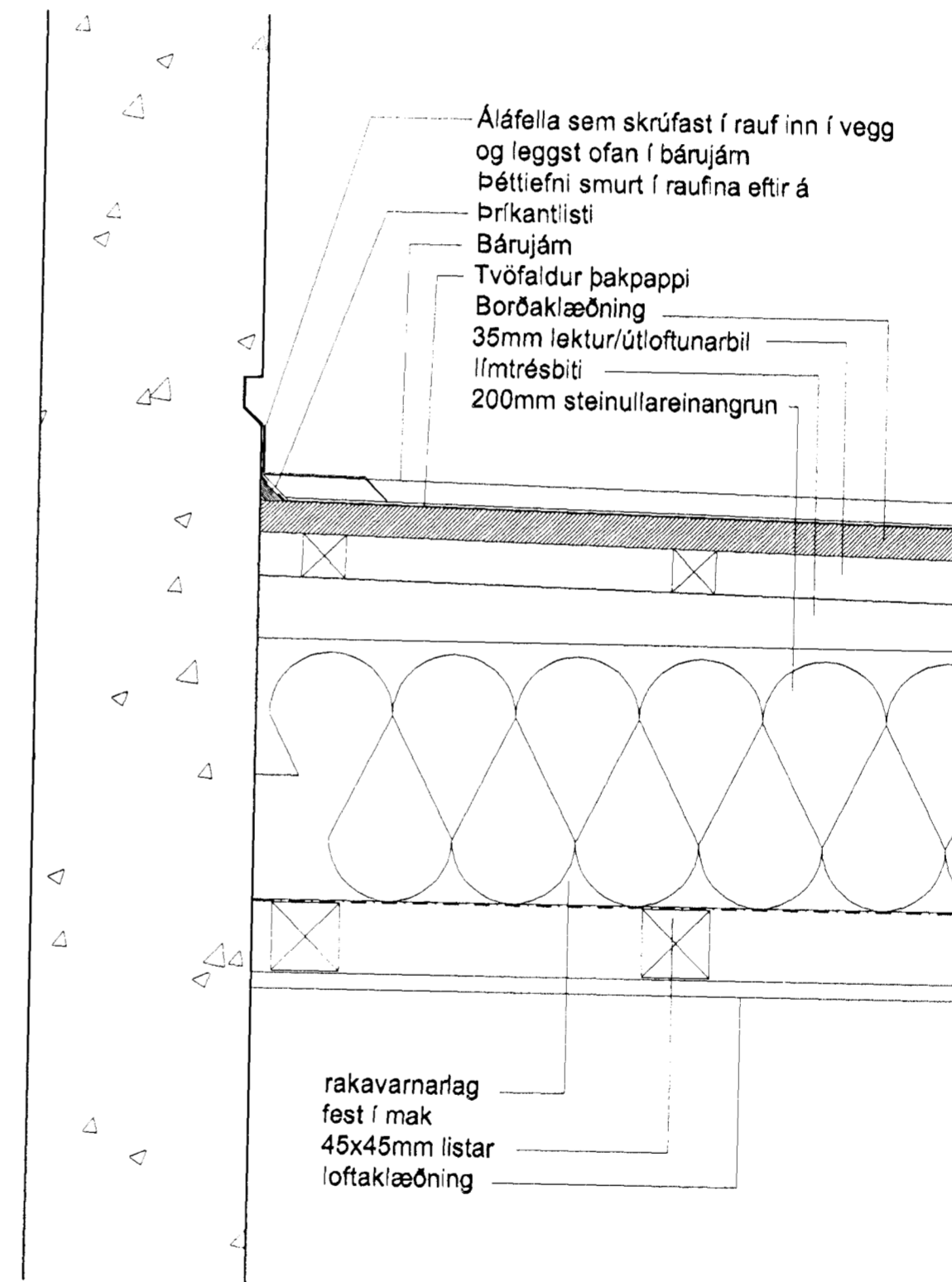
FRÁGANGUR MILLIÞAKS VIÐ STEYPTA VEGGI
