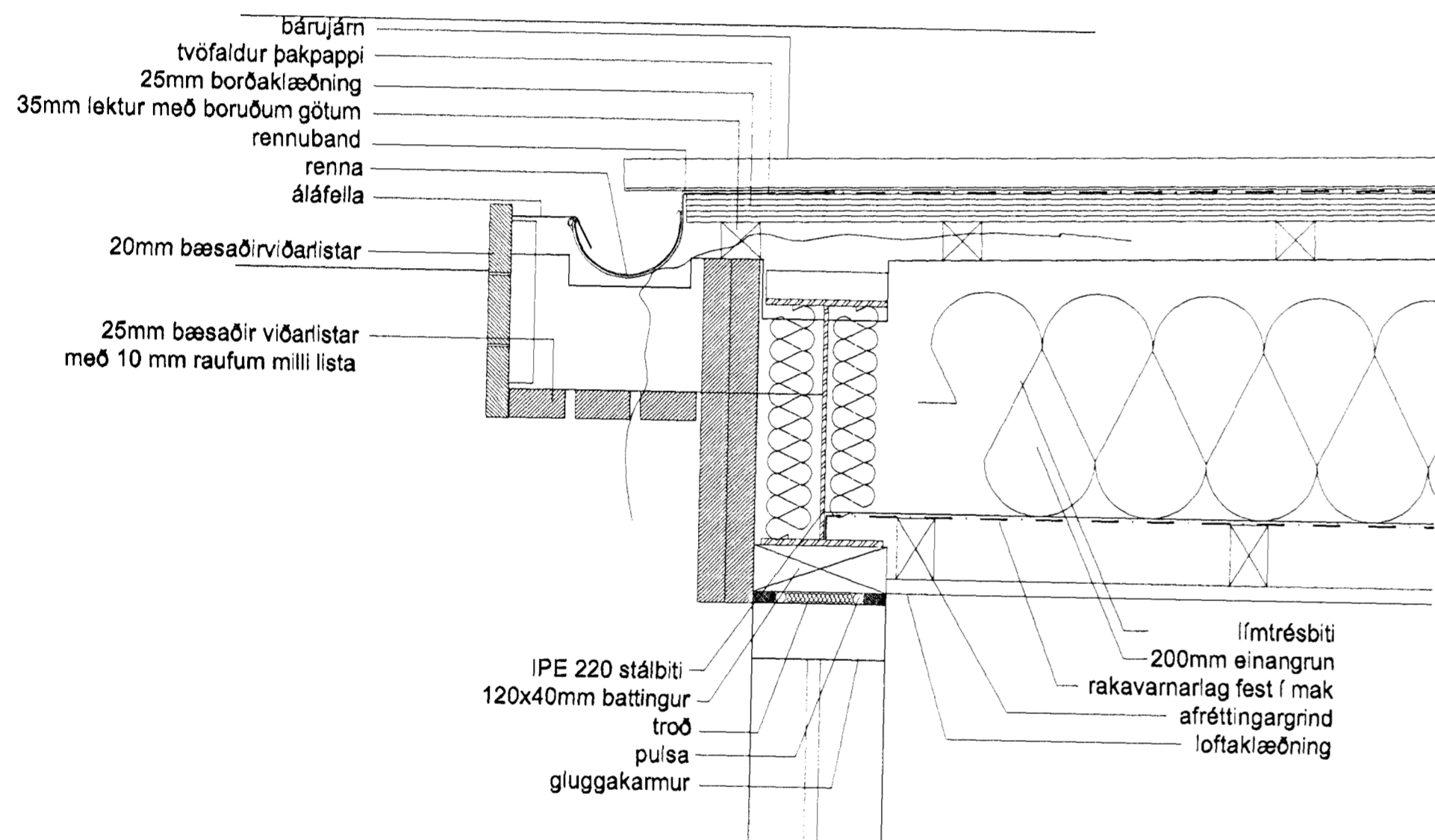
FRÁGANGUR VIÐ ÞAKKANT Á MILLIÞAKI
