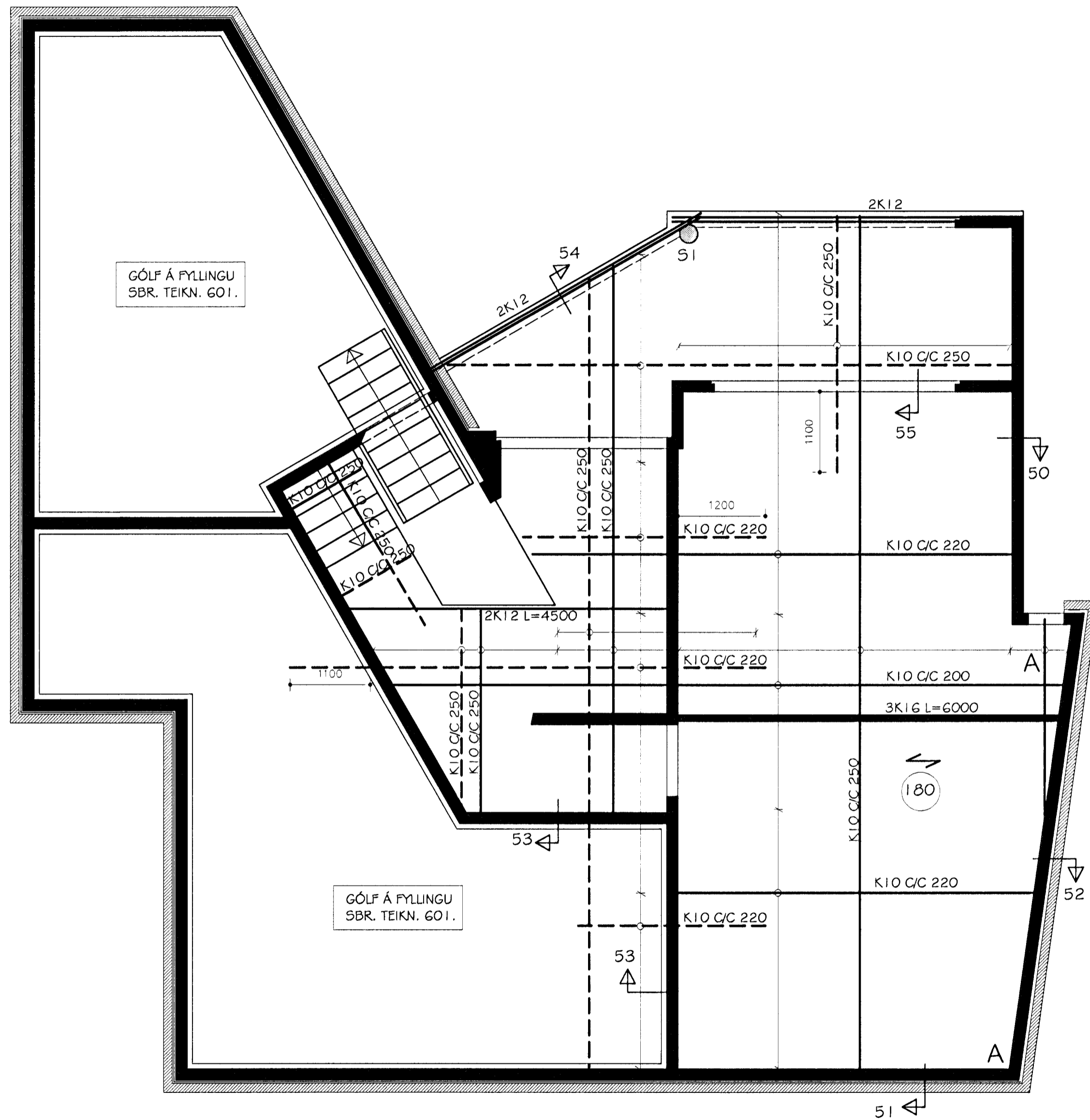
JÁRN Í PLÖTU YFIR NEDRI HÆÐ - GRUNNMYND MKV. 1:50
