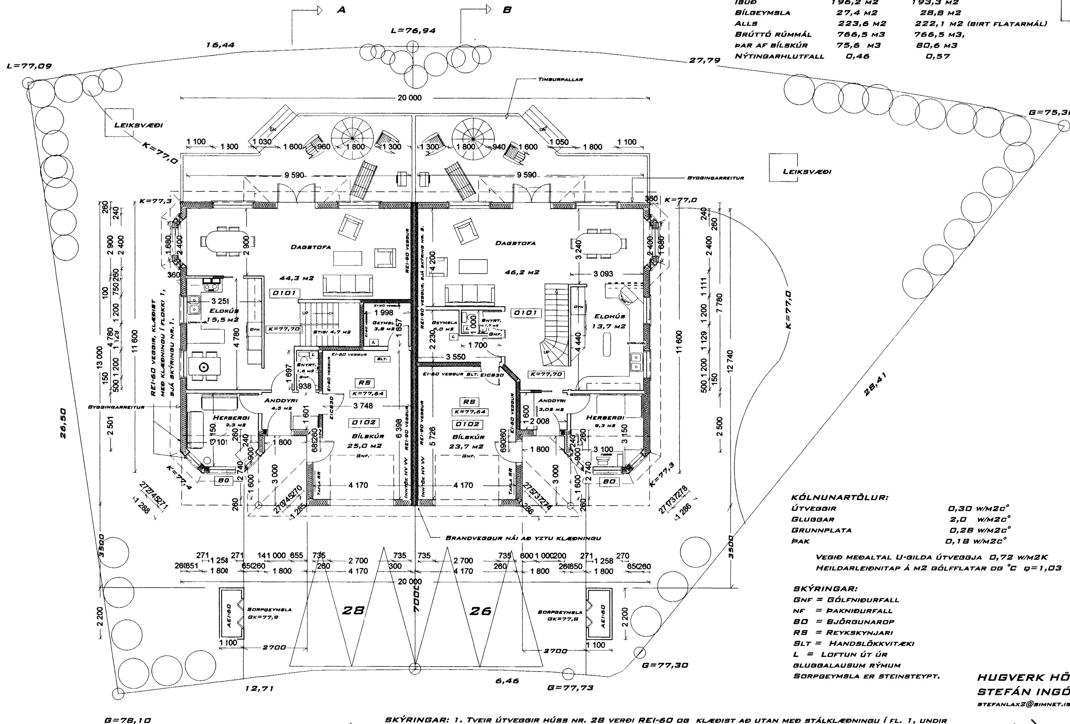
GRUNNMYND 1.HÆÐ, 1:100
