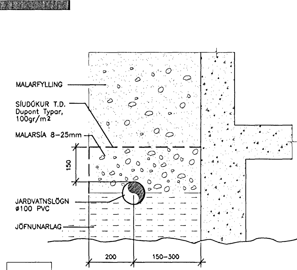
FRÁGANGUR JARÐVATNSLAGNA ÚR PVC M=1:20
