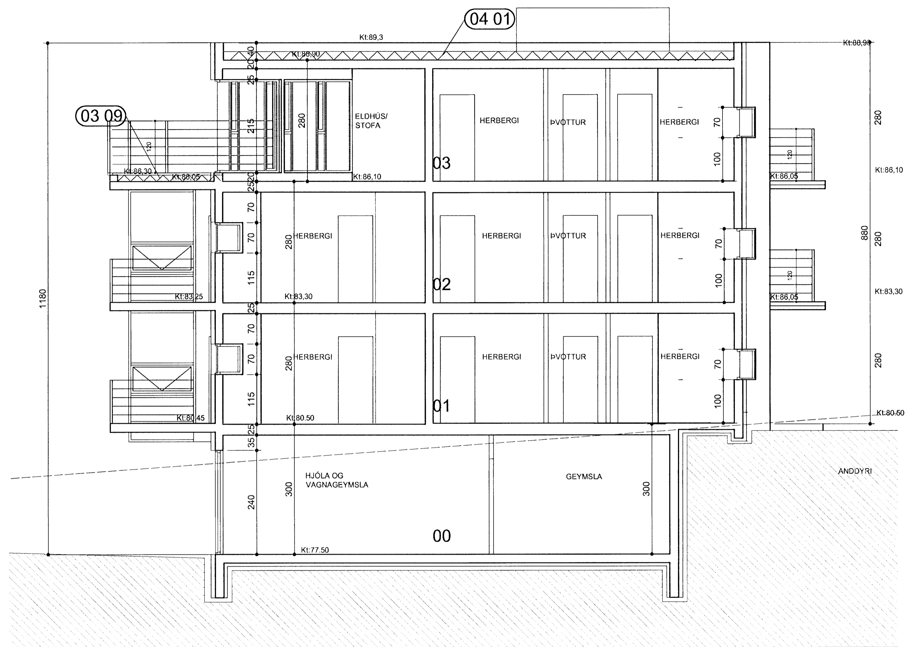
SNEIDING E-E
