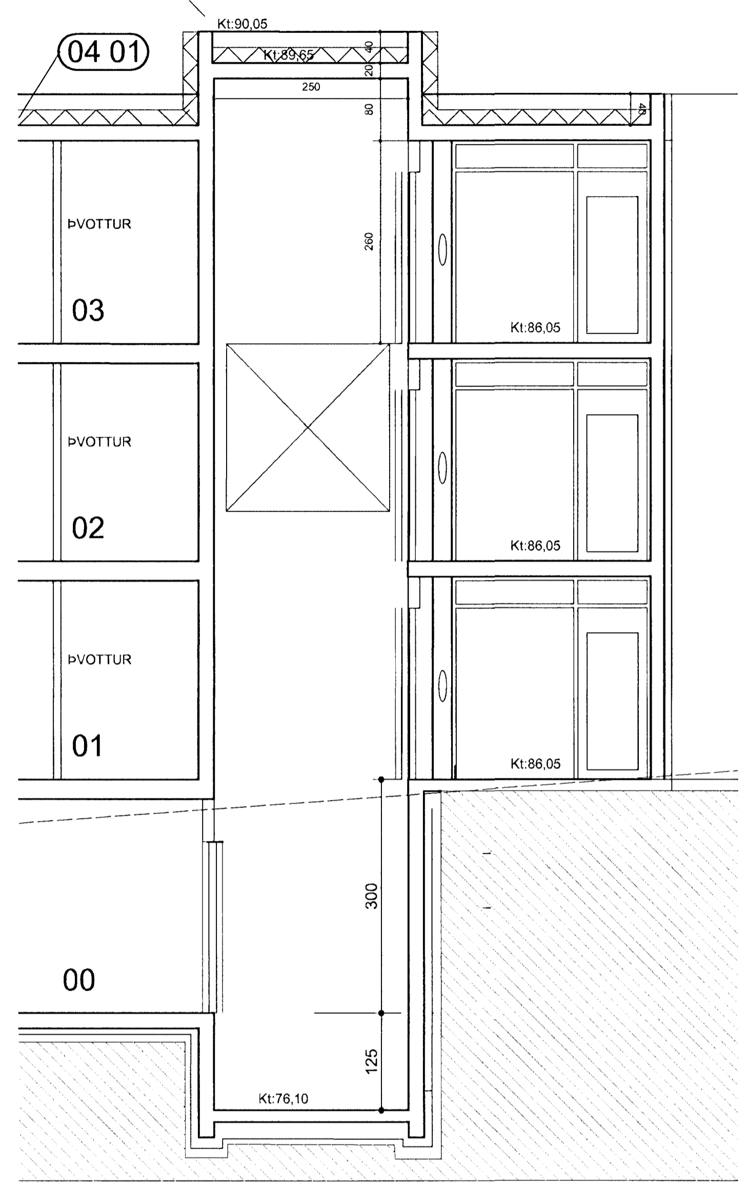
SNEIDING F-F
