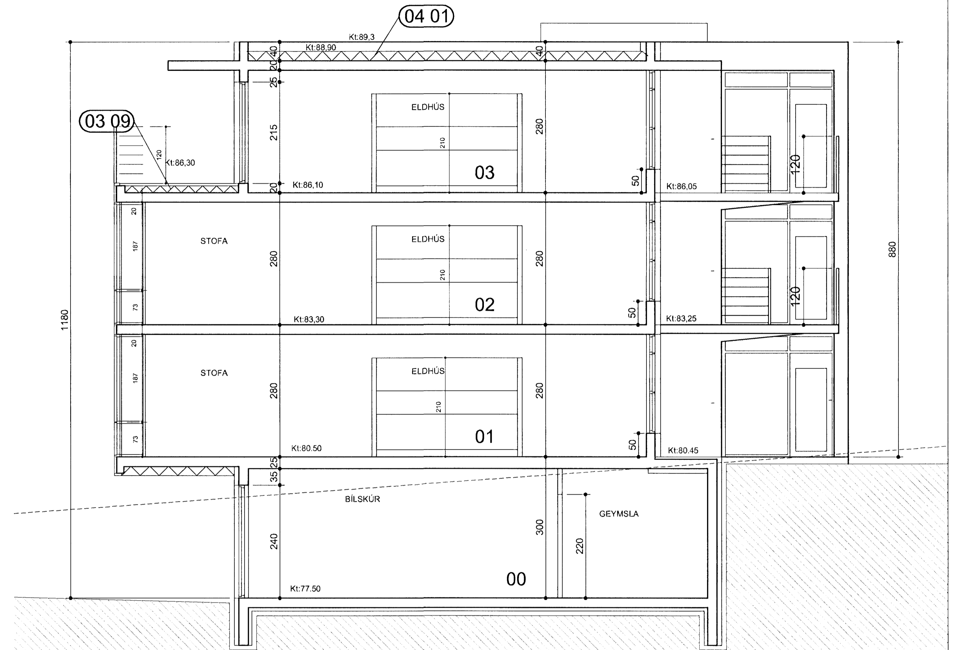
SNEIÐING D-D
